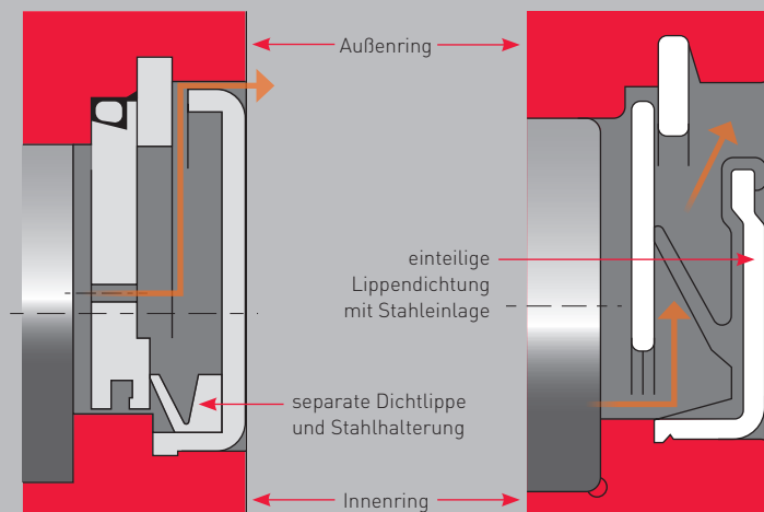
Öl-Luftstrom – Konventionell vs NSK Dichtungskonstruktion
