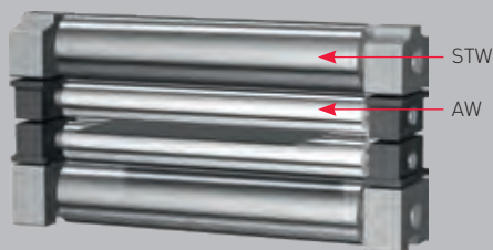
Tandem-Warmbandwalzwerk
