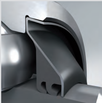
Zweilippendichtung
