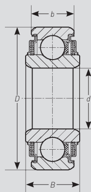
Rillenkugellager mit Zweilippendichtung
