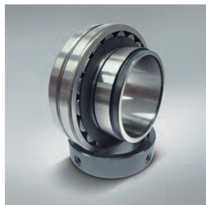
Ernte, Pendelrollenlager mit Exzenterring
