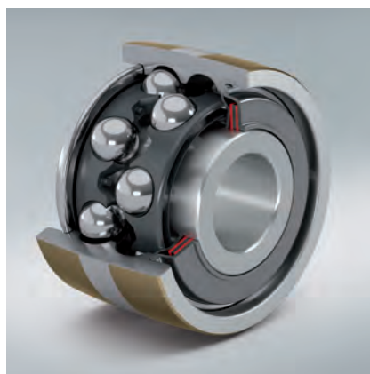
Futter, Stützrolle – zweireihig
