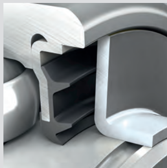
Dreilippendichtung
