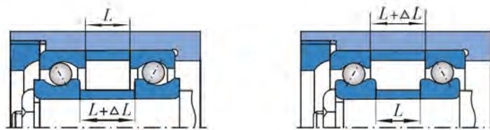
Fig. 13 Position preload
