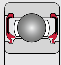
DDW Leichtkontakt Dichtscheibe
