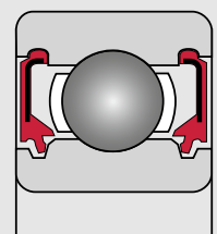
DDU schleifende Dichtscheibe
