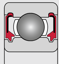
VV nicht schleifende Dichtscheibe
