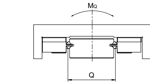
Zulässige Momente Typ SK und SKD
