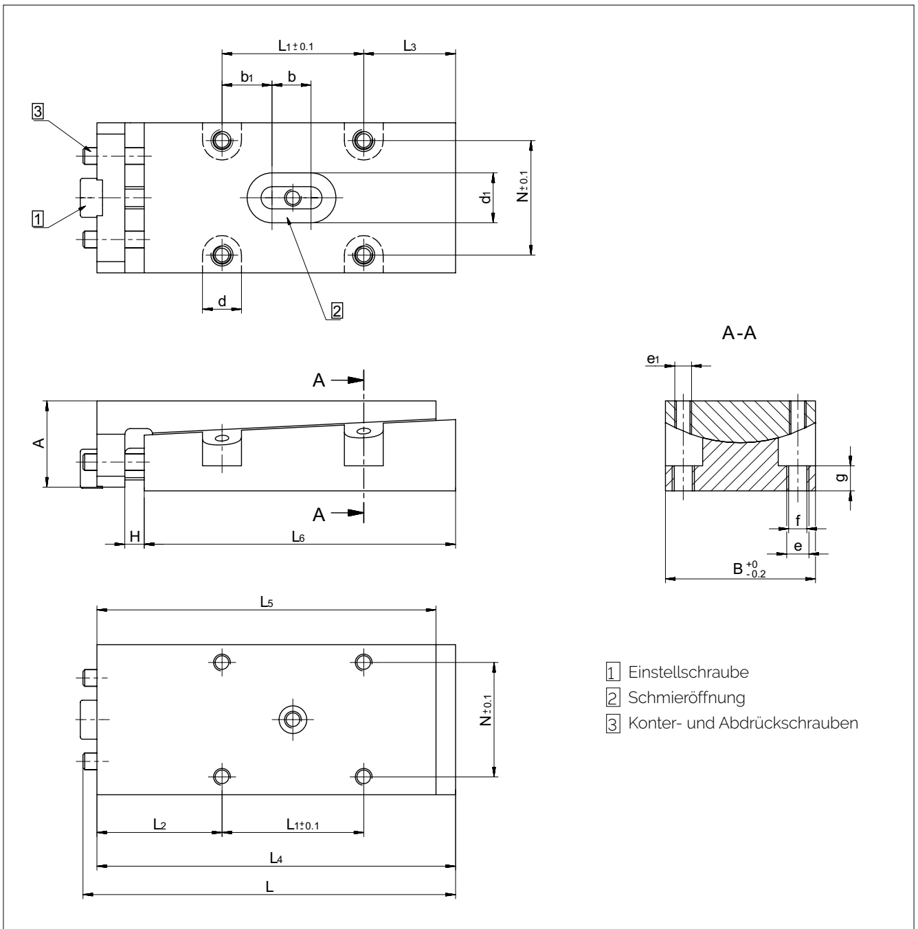
Vorspannkeil NRV
