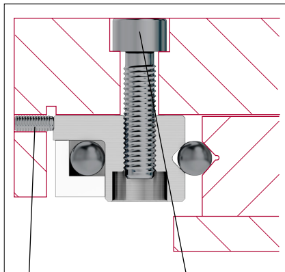
Stellschrauben Befestigungsschrauben
