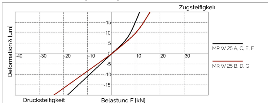
AMSABS 3L W 25 Steifigkeitsdiagramm
