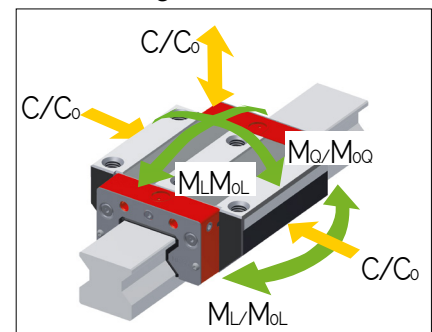
MR W 65 Tragzahlen
