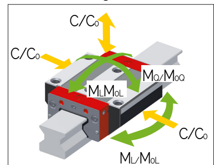
AMS 3B W 25 Tragzahlen
