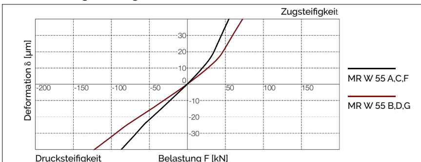
MR W 55 Steifigkeitsdiagramm
