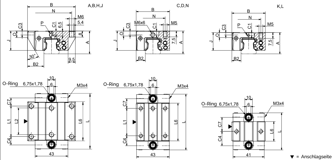
BM W 20 Masszeichnungen
