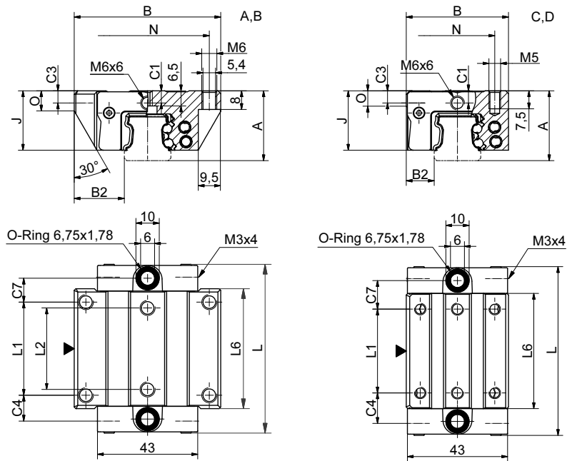
BM WR 20 Masszeichnungen
