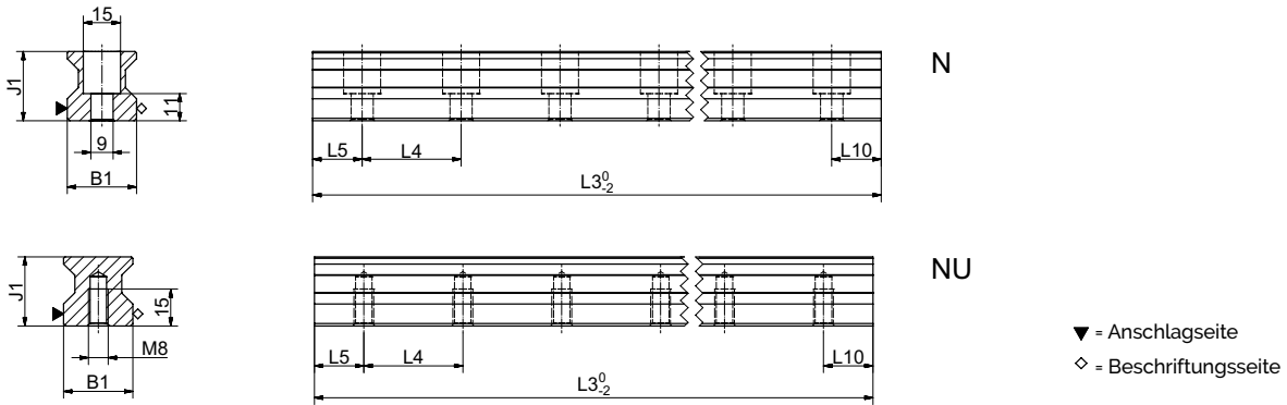
MR S 30 Masszeichnungen
