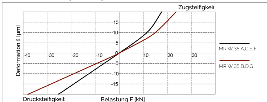
AMS 3B W 35 Steifigkeitsdiagramm
