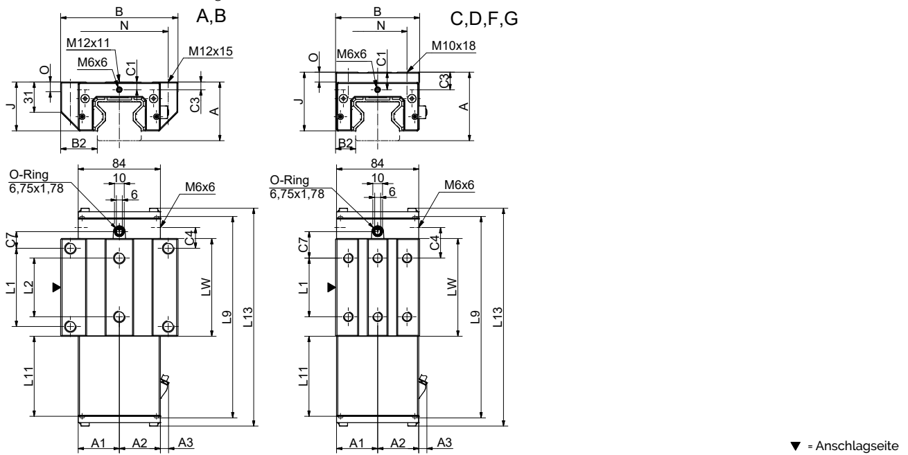
AMS 3B W 45 Masszeichnungen
