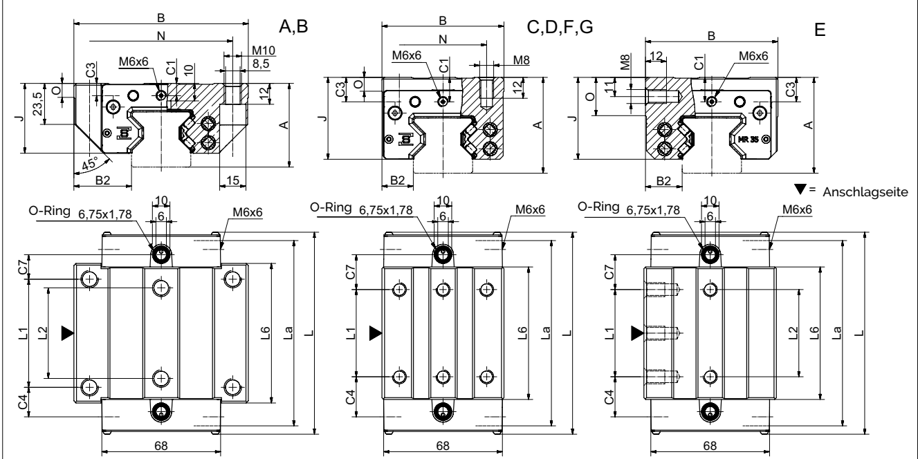
MR W 35 Masszeichnungen
