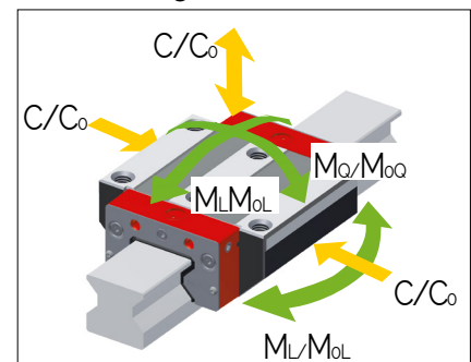
MR W 30 Tragzahlen
