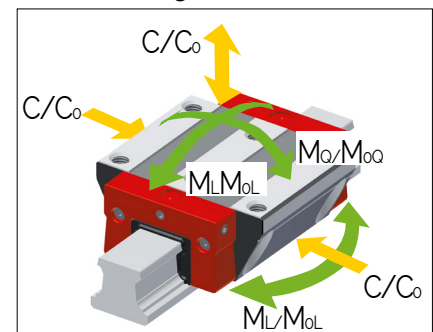
BM WR 35 Tragzahlen
