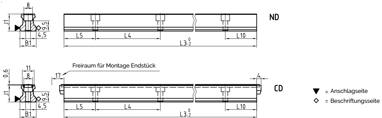
AMS 4B S 15 Masszeichnungen
