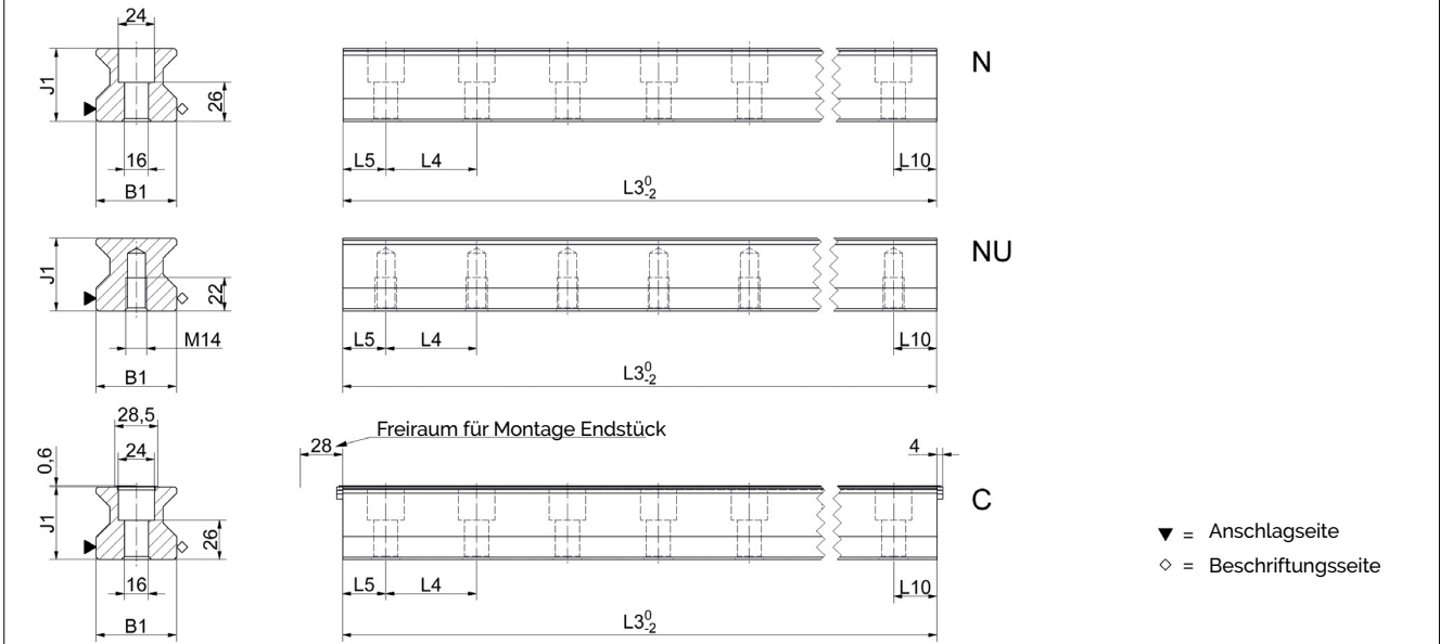
MR S 55 Masszeichnungen
