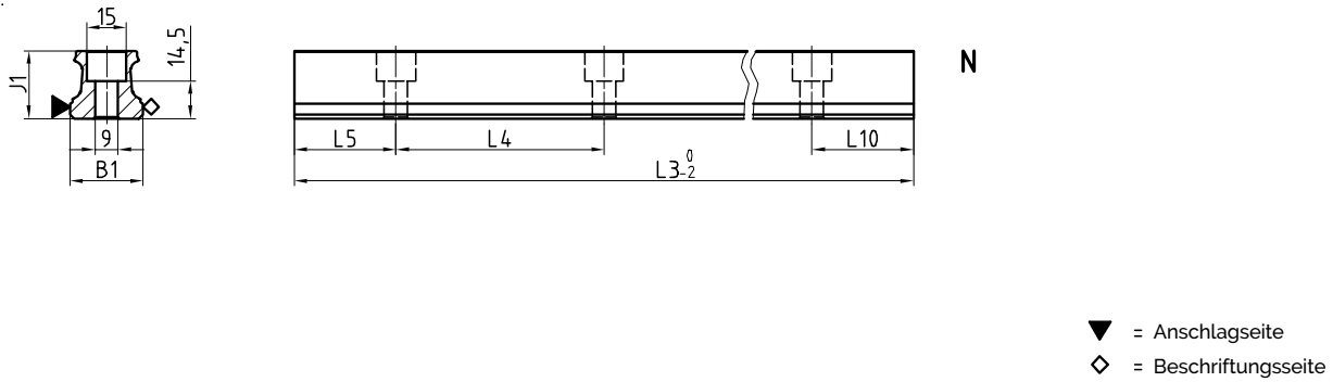
AMS 4B S 30 Masszeichnungen
