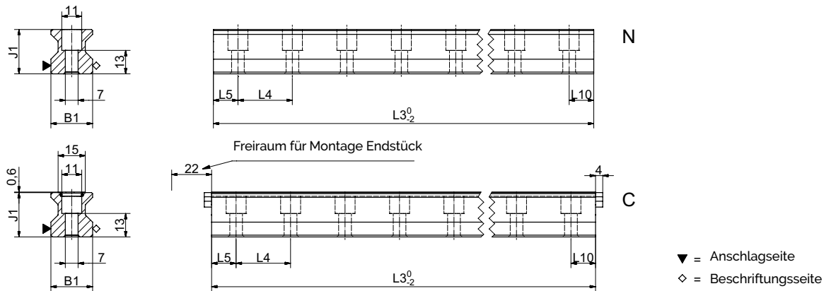
AMS 3B S 25 Masszeichnungen
