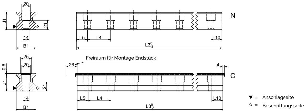
AMSABS 3B S 45 Masszeichnungen
