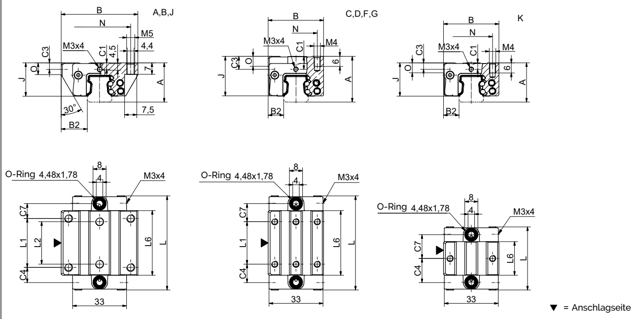
BM W 15 Masszeichnungen
