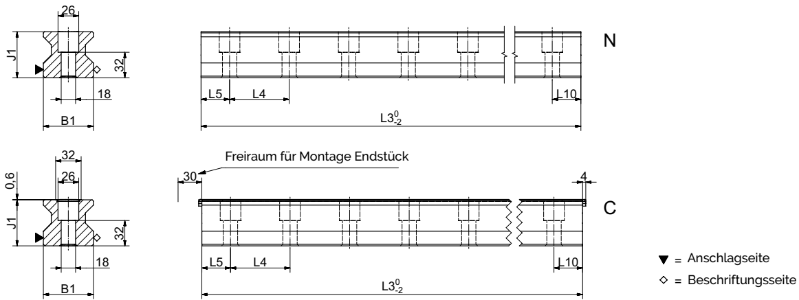
AMSABS 3B S 65 Masszeichnungen
