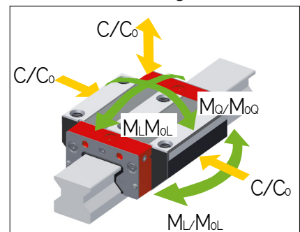
AMSABS 3B W 55 Tragzahlen
