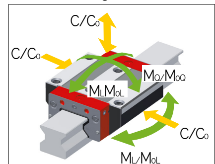
AMS 4B W 15 Tragzahlen
