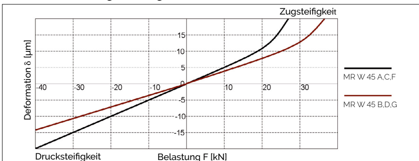
AMS 3B W 45 Steifigkeitsdiagramm
