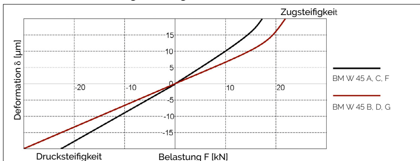
AMSABS 4B W 45 Steifigkeitsdiagramm
