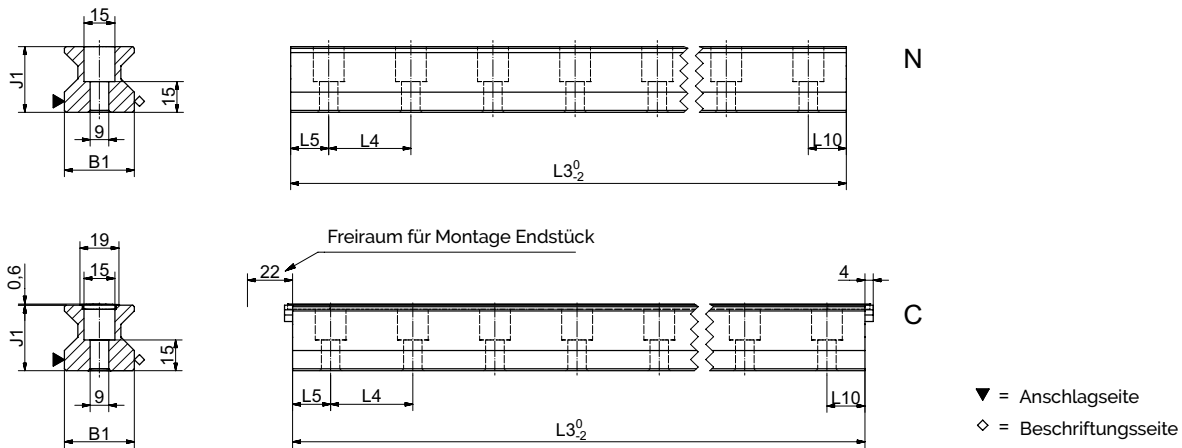
AMSABS 3B S 35 Masszeichnungen
