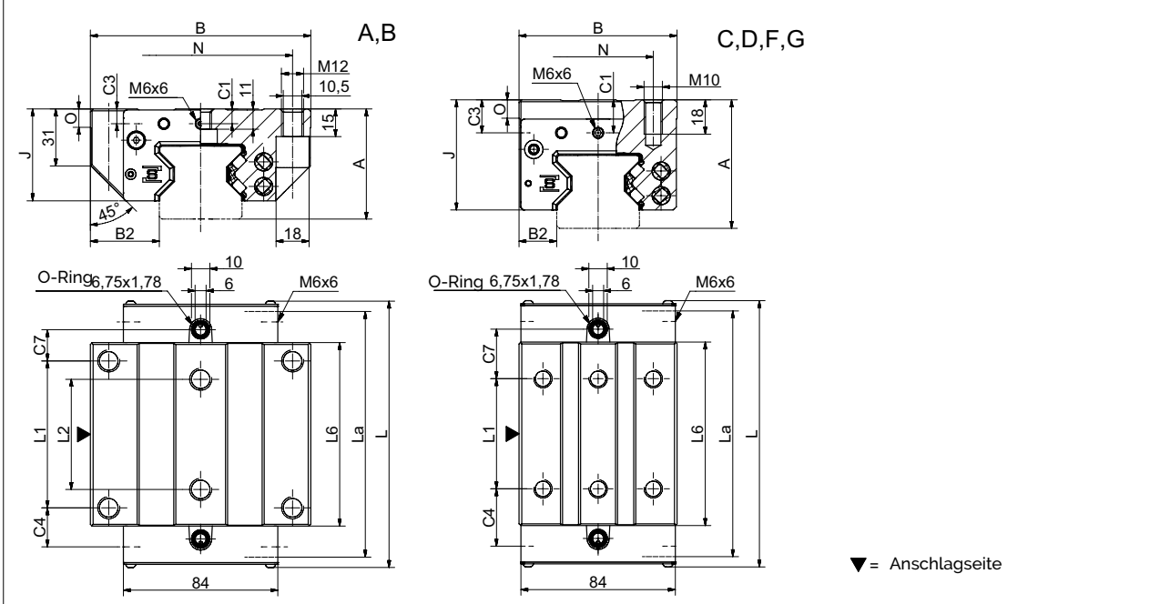
MR W 45 Masszeichnungen
