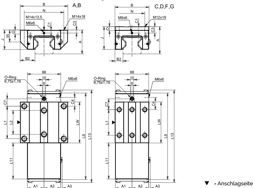
AMSABS 3B W 55 Masszeichnungen
