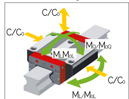
AMSABS 3B W 45 Tragzahlen
