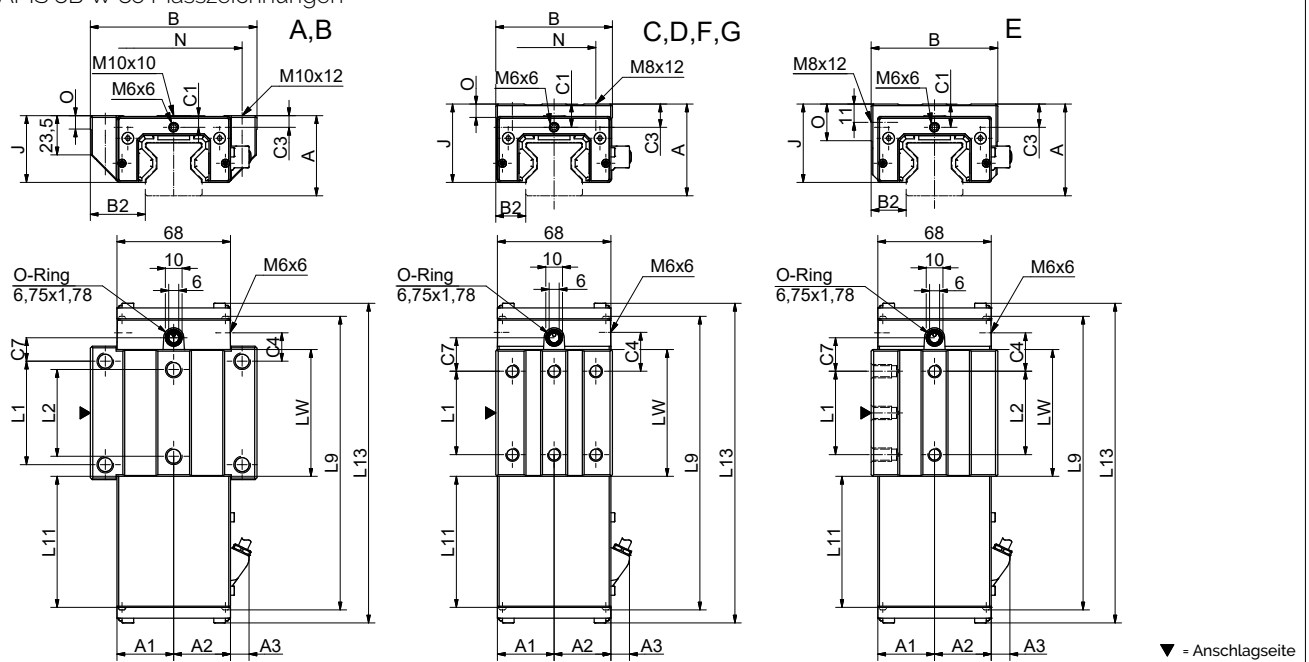
AMS 3B W 35 Masszeichnungen
