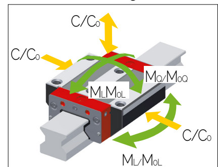
AMSABS 3L W 25 Tragzahlen
