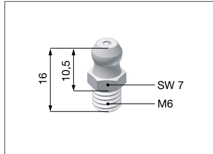
Schmiernippel SN 6 Kegelschmiernippel gerade
