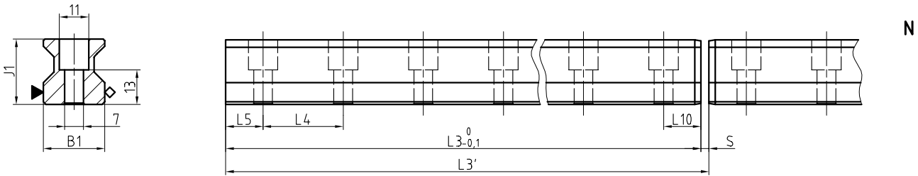
AMSABS 3L S 25 Masszeichnungen
