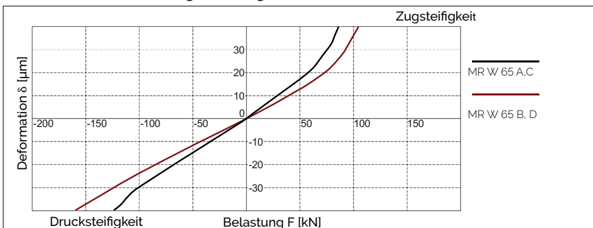
AMSABS 3L W 65 Steifigkeitsdiagramm
