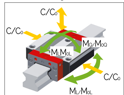
AMS 4B W 30 Tragzahlen
