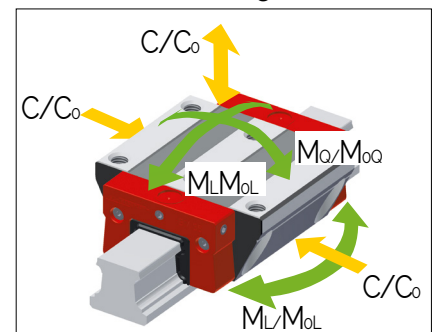
AMSABS 4B W 30 Tragzahlen
