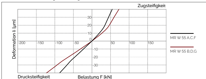
AMS 3B W 55 Steifigkeitsdiagramm
