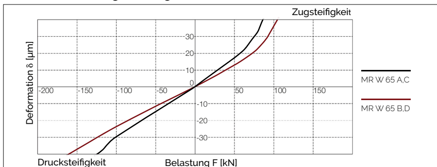
AMS 3B W 65 Steifigkeitsdiagramm
