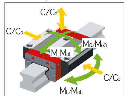
MR W 55 Tragzahlen
