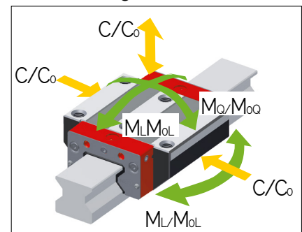
MR W 100 Tragzahlen
