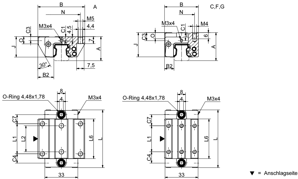
BM WR 15 Masszeichnungen
