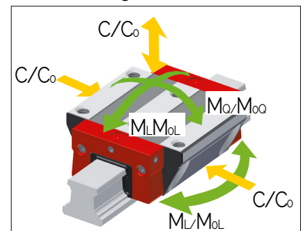
BM WR 25 Tragzahlen
