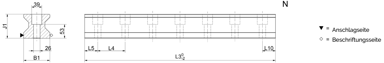
MR S 100 Masszeichnungen
