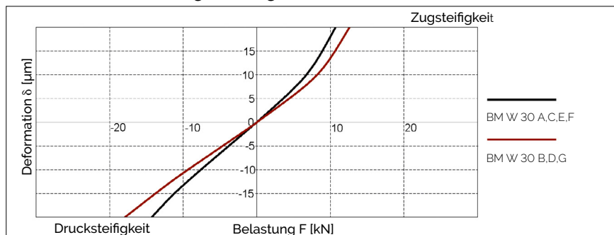
AMSABS 4B W 30 Steifigkeitsdiagramm
