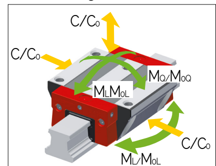
BM WR 30 Tragzahlen
