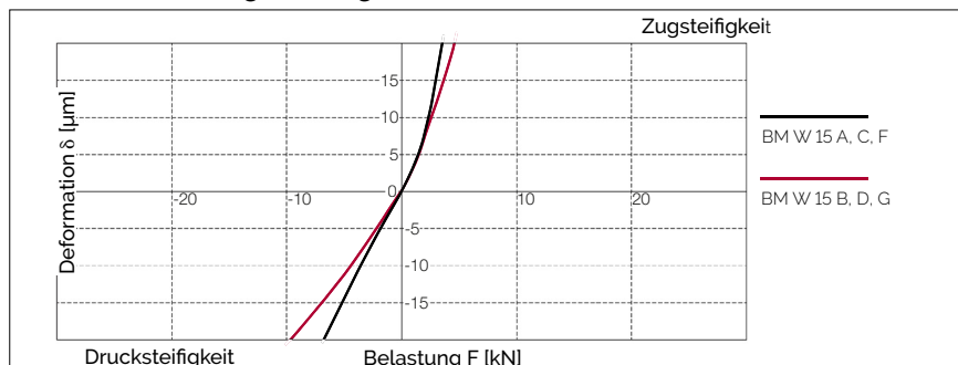
AMS 4B W 15 Steifigkeitsdiagramm
