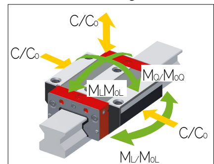
AMSABS 3L W 30 Tragzahlen
