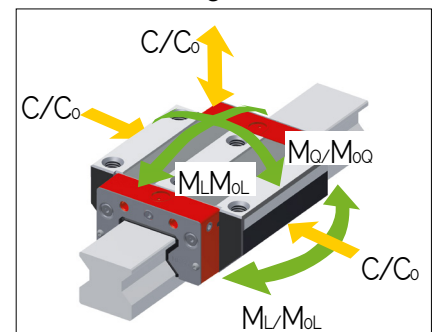
AMS 3B W 35 Tragzahlen
