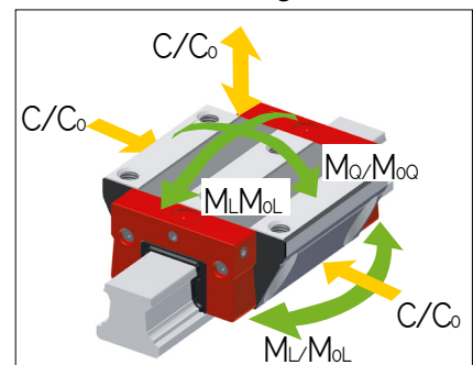
AMSABS 4B W 45 Tragzahlen
