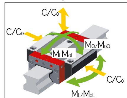
AMS 3B W 45 Tragzahlen
