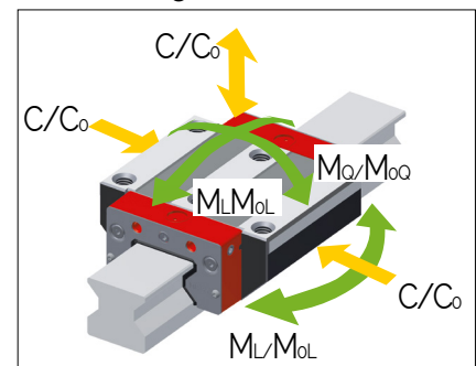
MR W 35 Tragzahlen
