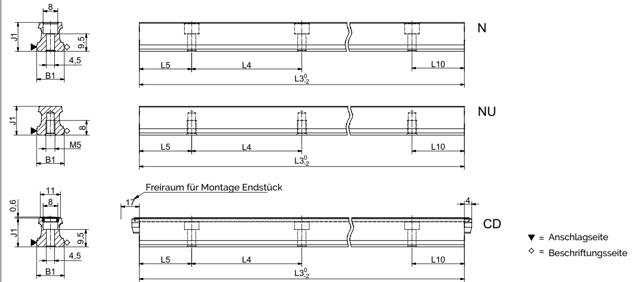
BM S 15 Masszeichnungen
