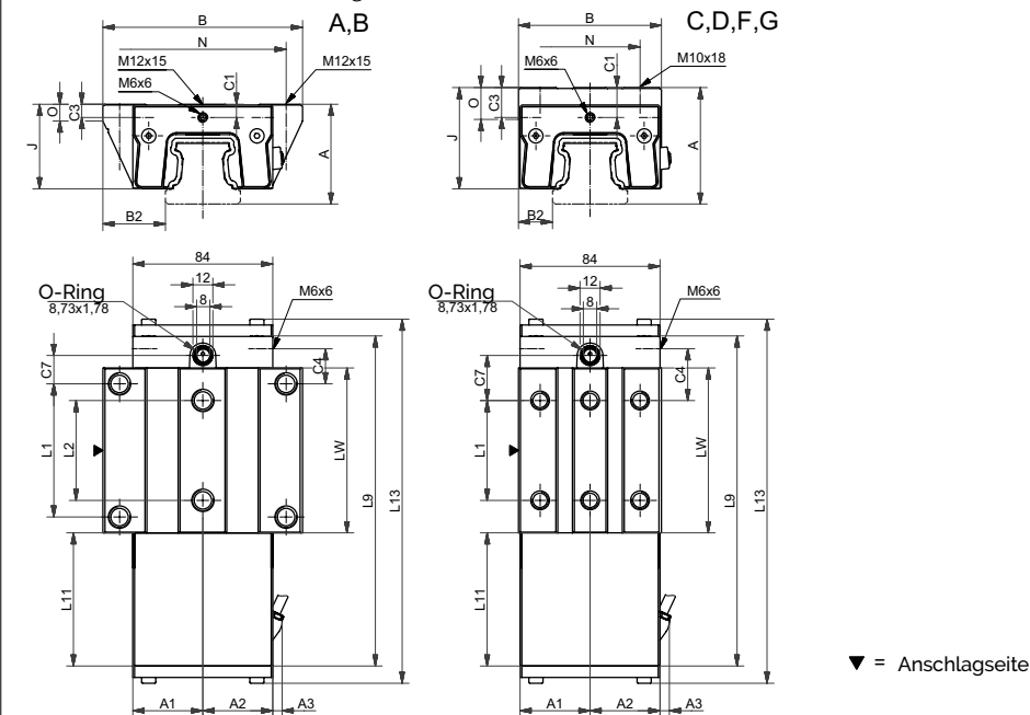
AMS 4B W 45 Masszeichnungen
