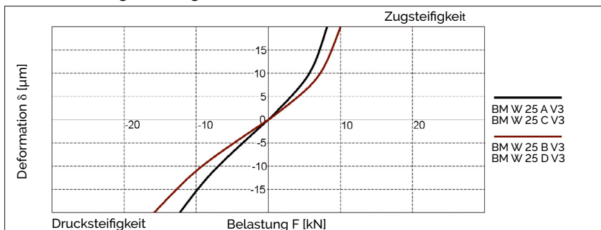
BM W 25 Steifigkeitsdiagramm
