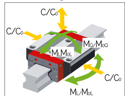
AMS 3B W 55 Tragzahlen
