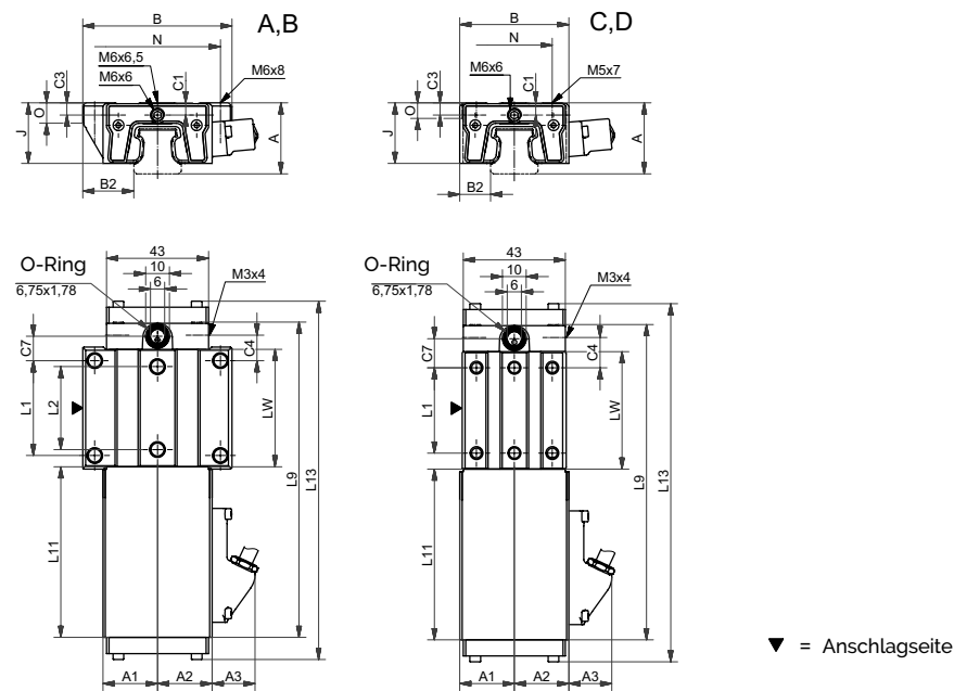
AMS 4B W 20 Masszeichnungen
