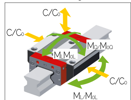
AMSABS 3L W 45 Tragzahlen
