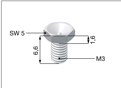
Schmiernippel SN 3-T Trichterschmiernippel M3
