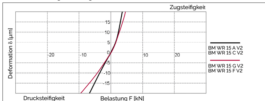
BM WR 15 Steifigkeitsdiagramm
