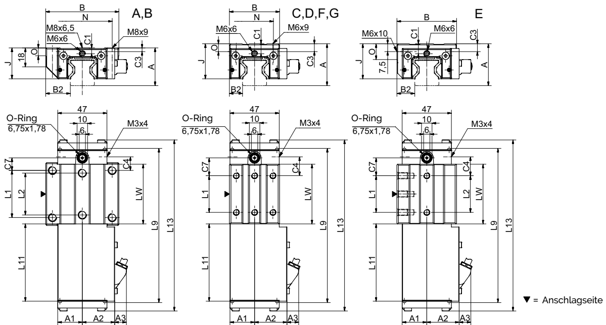
AMS 3B W 25 Masszeichnungen
