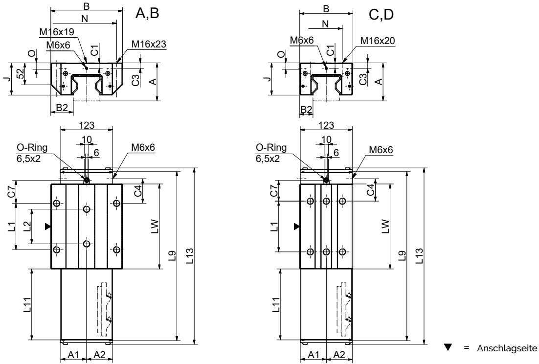
AMSABS 3L W 65 Masszeichnungen
