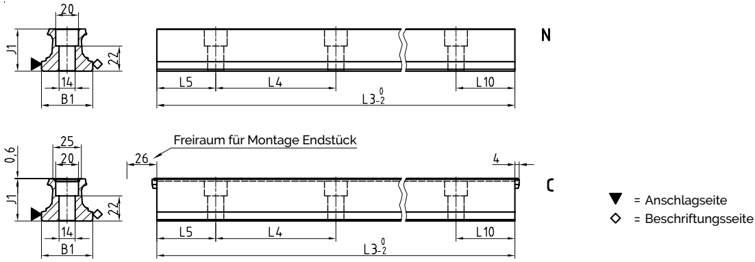
AMSABS 4B S 45 Masszeichnungen
