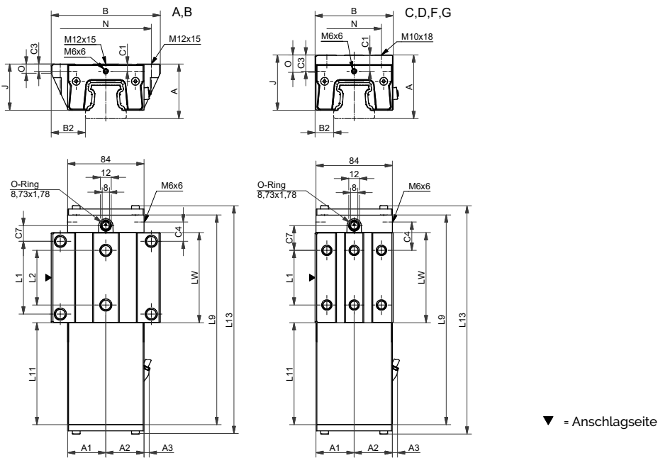
AMSABS 4B W 45 Masszeichnungen
