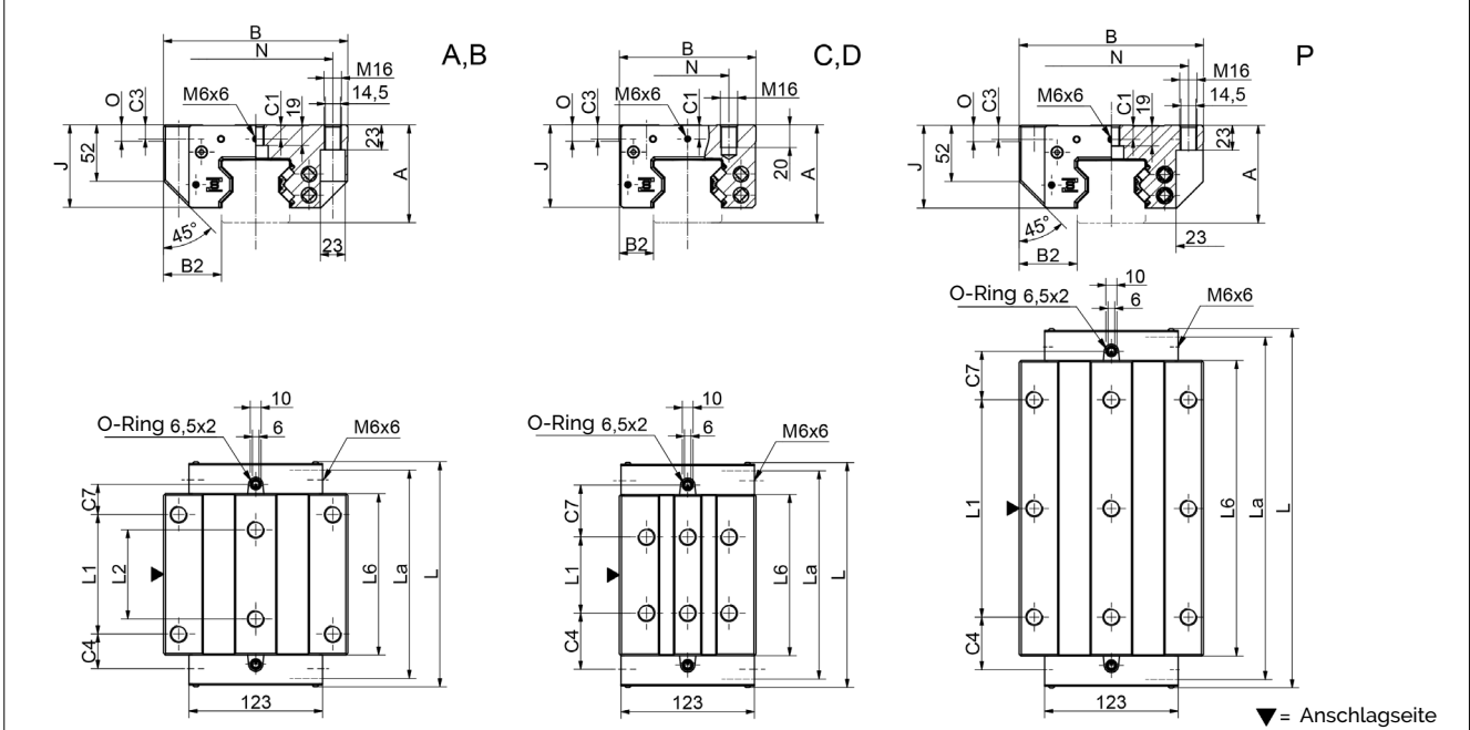
MR W 65 Masszeichnungen
