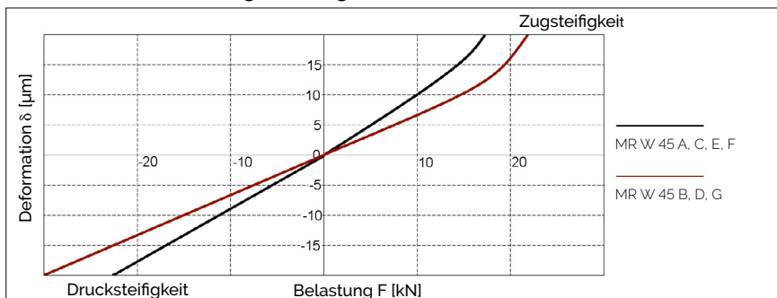
AMSABS 3L W 45 Steifigkeitsdiagramm
