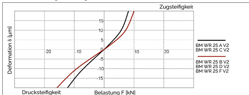
BM WR 25 Steifigkeitsdiagramm
