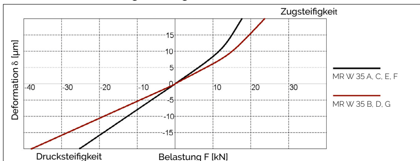
AMSABS 3L W 35 Steifigkeitsdiagramm
