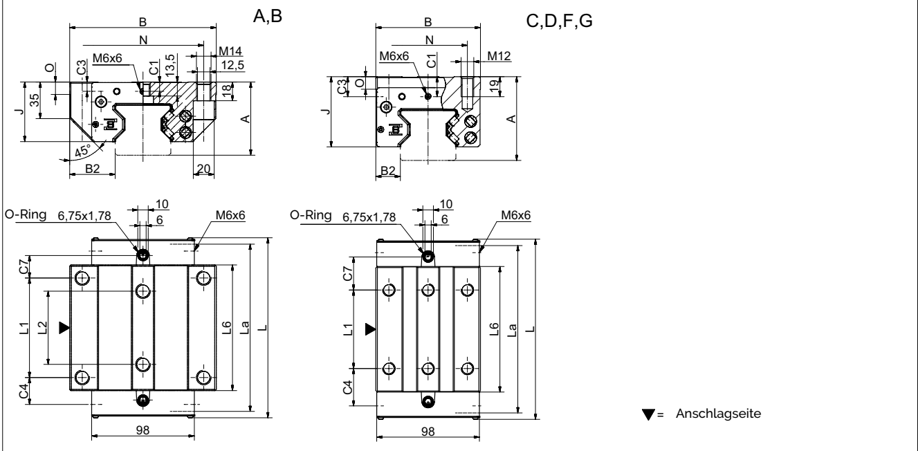
MR W 55 Masszeichnungen
