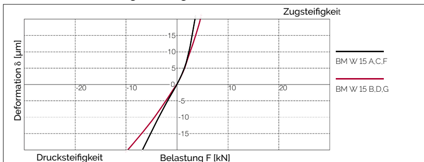
AMSABS 4B W 15 Steifigkeitsdiagramm
