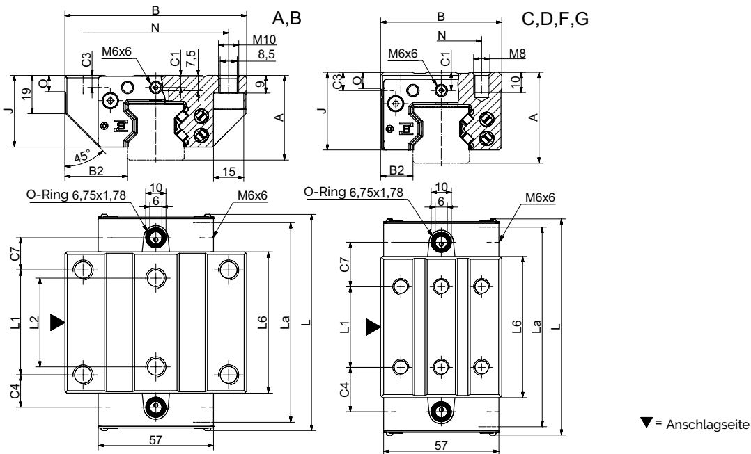
MR W 30 Masszeichnungen
