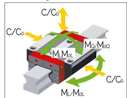
MR W 45 Tragzahlen
