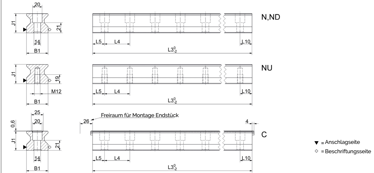
MR S 45 Masszeichnungen
