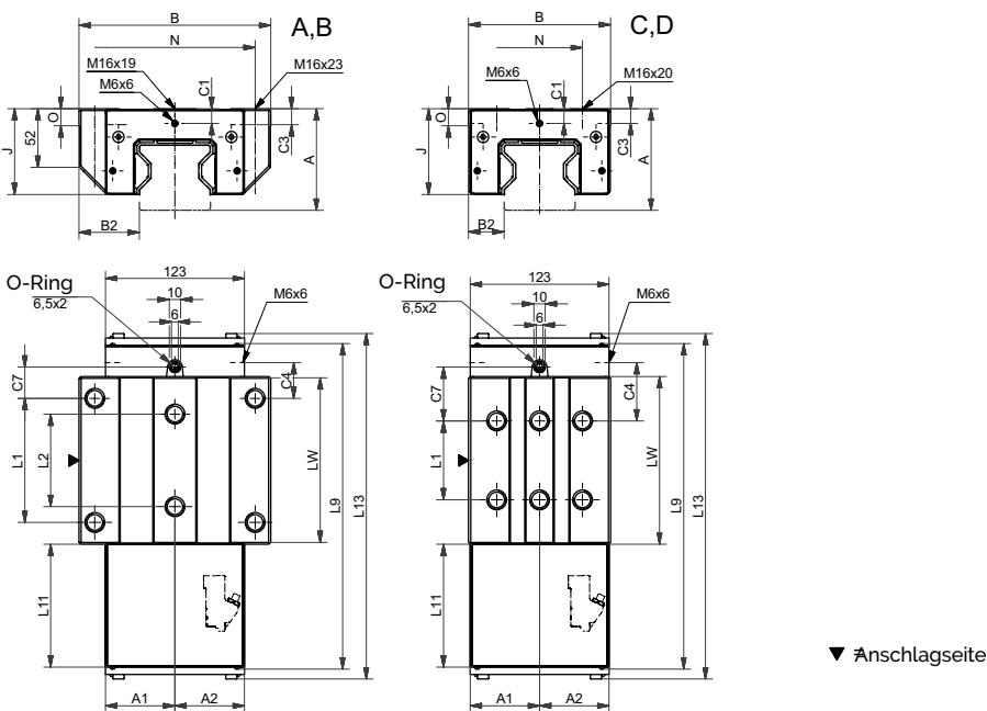
AMSABS 3B W 65 Masszeichnungen
