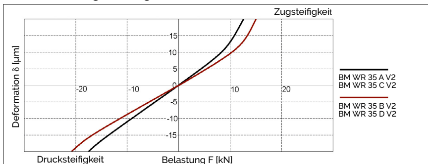
BM WR 35 Steifigkeitsdiagramm
