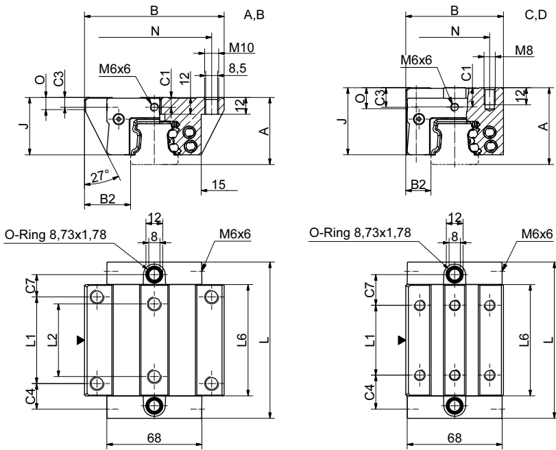
BM WR 35 Masszeichnungen
