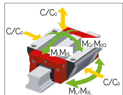
BM W 15 Tragzahlen
