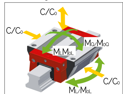
BM W 25 Tragzahlen
