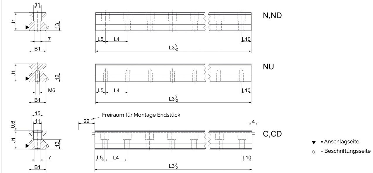
MR S 25 Masszeichnungen
