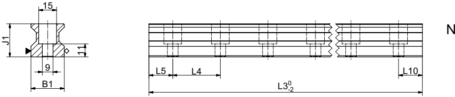
AMS 3B S 30 Masszeichnungen
