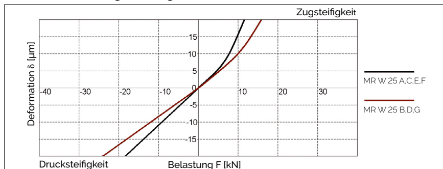
AMS 3B W 25 Steifigkeitsdiagramm
