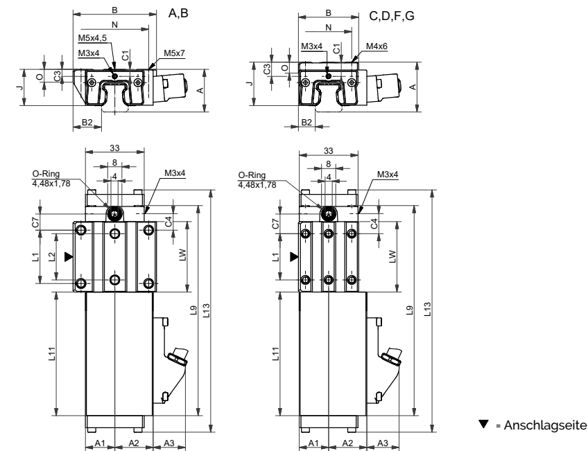
AMS 4B W 15 Masszeichnungen
