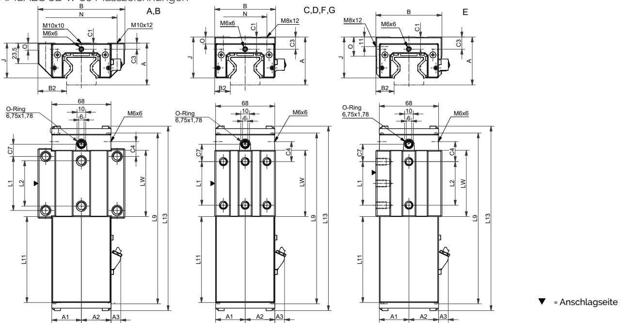
AMSABS 3B W 35 Masszeichnungen
