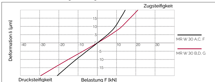
AMSABS 3L W 30 Steifigkeitsdiagramm
