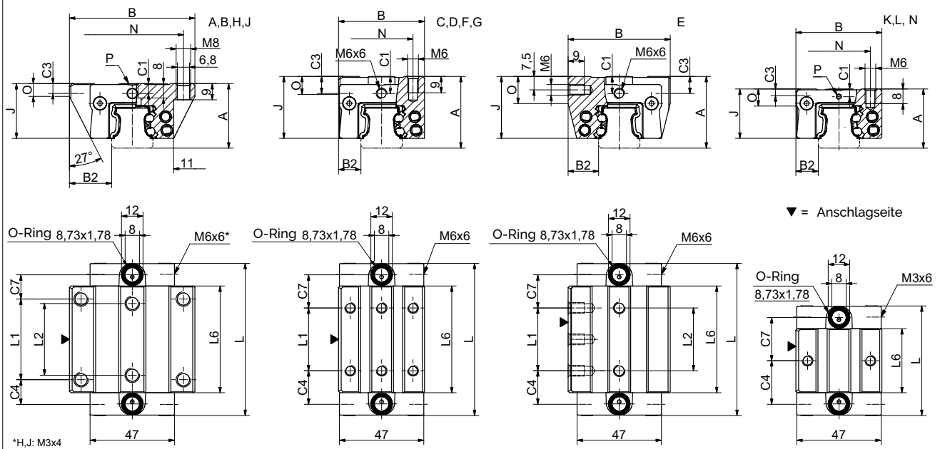
BM W 25 Masszeichnungen
