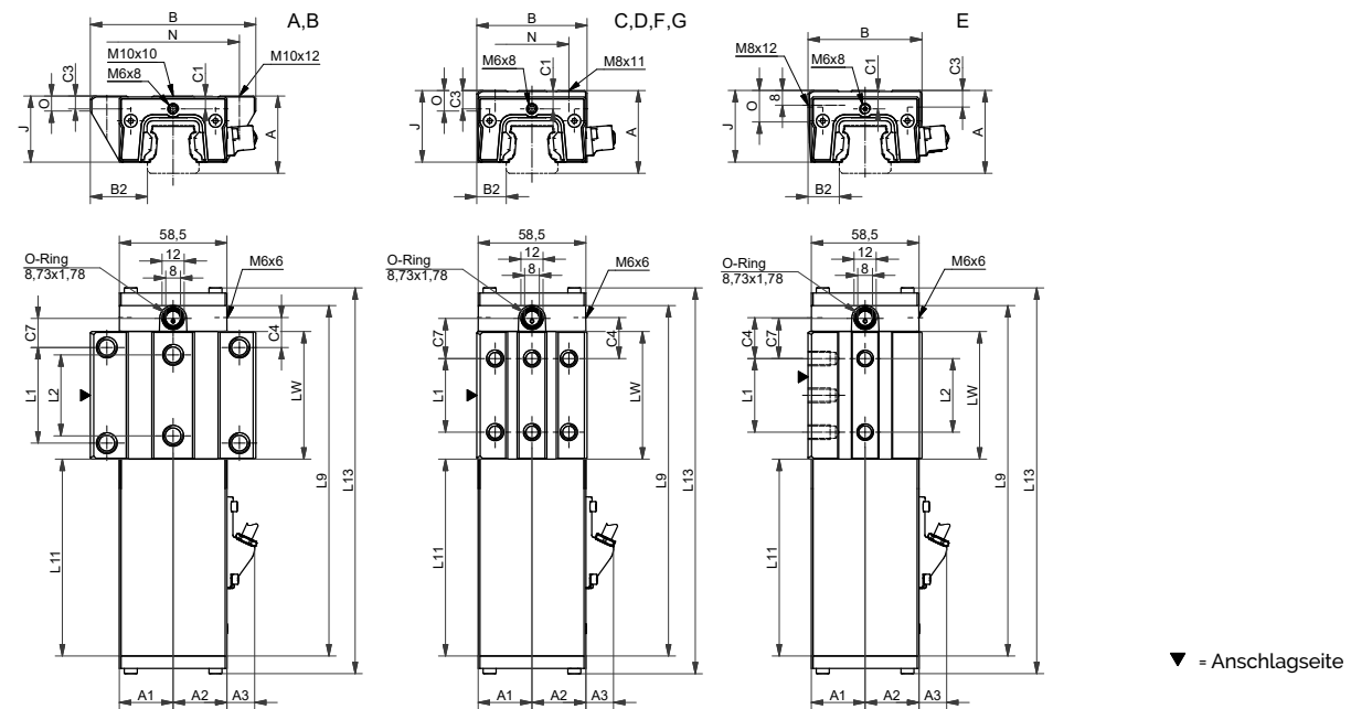
AMSABS 4B W 30 Masszeichnungen
