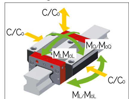
MR W 25 Tragzahlen
