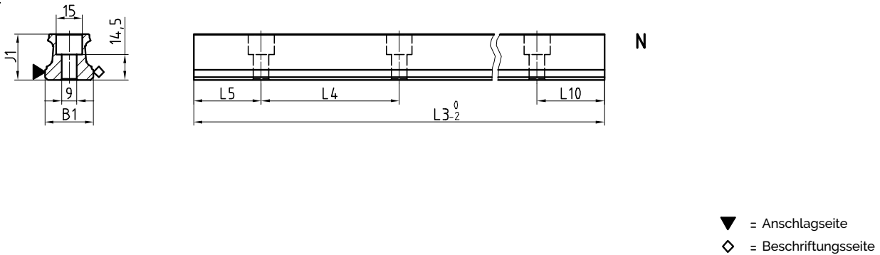
AMSABS 4B S 30 Masszeichnungen
