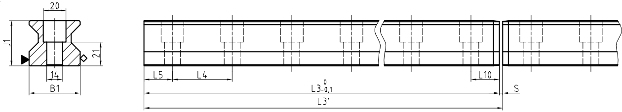
AMSABS 3L S 45 Masszeichnungen
