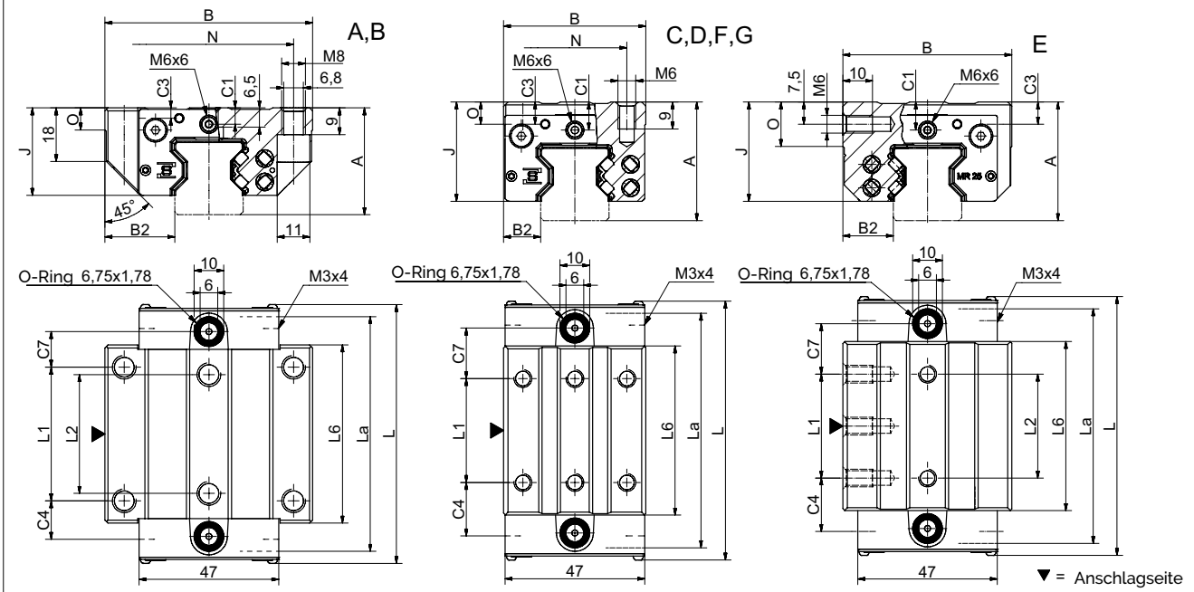
MR W 25 Masszeichnungen
