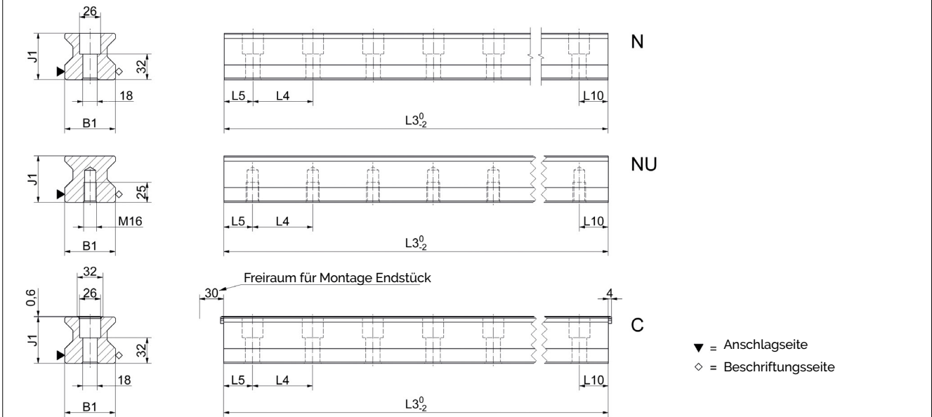
MR S 65 Masszeichnungen
