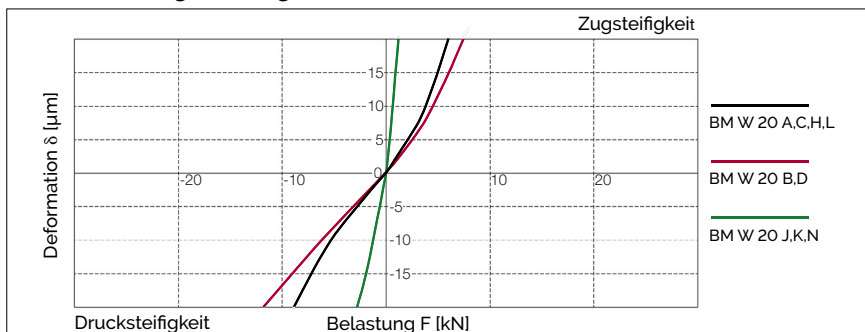
BM W 20 Steifigkeitsdiagramm
