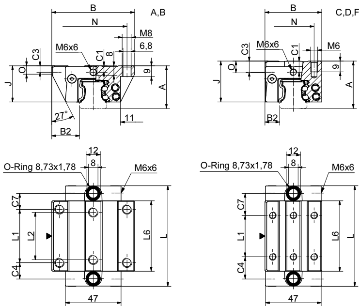
BM WR 25 Masszeichnungen
