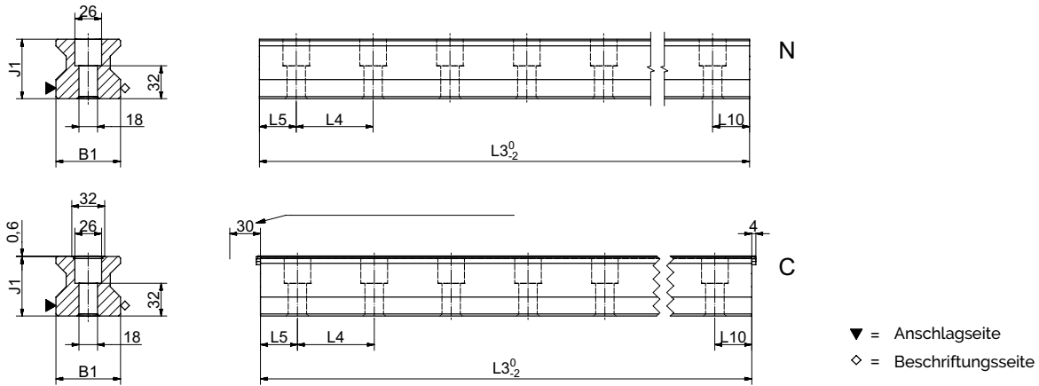
AMS 3B S 65 Masszeichnungen
