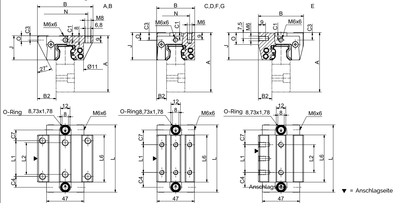
BM W 25 Masszeichnungen - BZ
