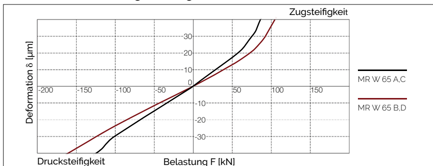
AMSABS 3B W 65 Steifigkeitsdiagramm
