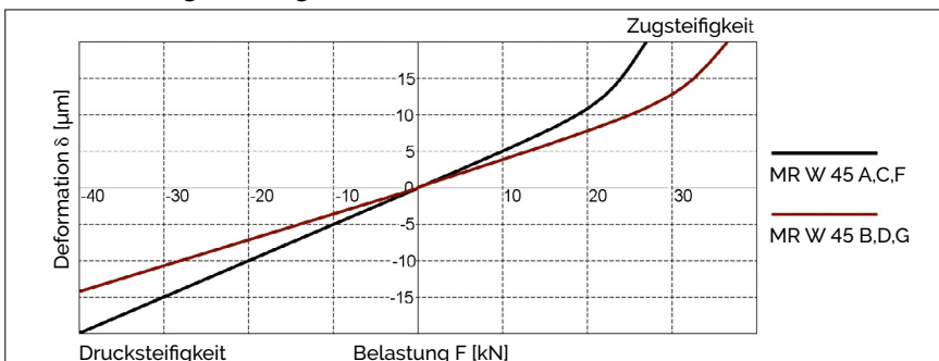
MR W 45 Steifigkeitsdiagramm
