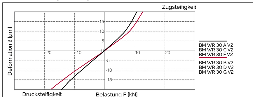
BM WR 30 Steifigkeitsdiagramm
