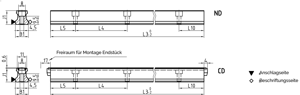
AMSABS 4B S 15 Masszeichnungen
