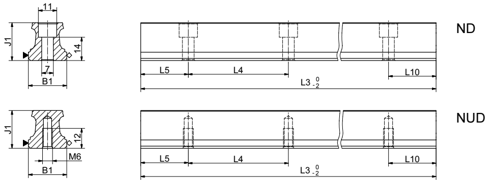
BM SR 25 Masszeichnungen
