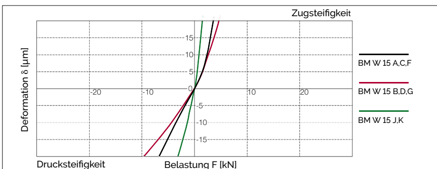
BM W 15 Steifigkeitsdiagramm
