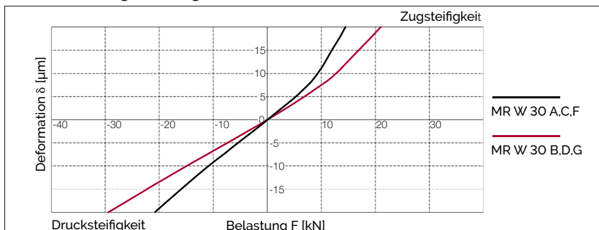
MR W 30 Steifigkeitsdiagramm
