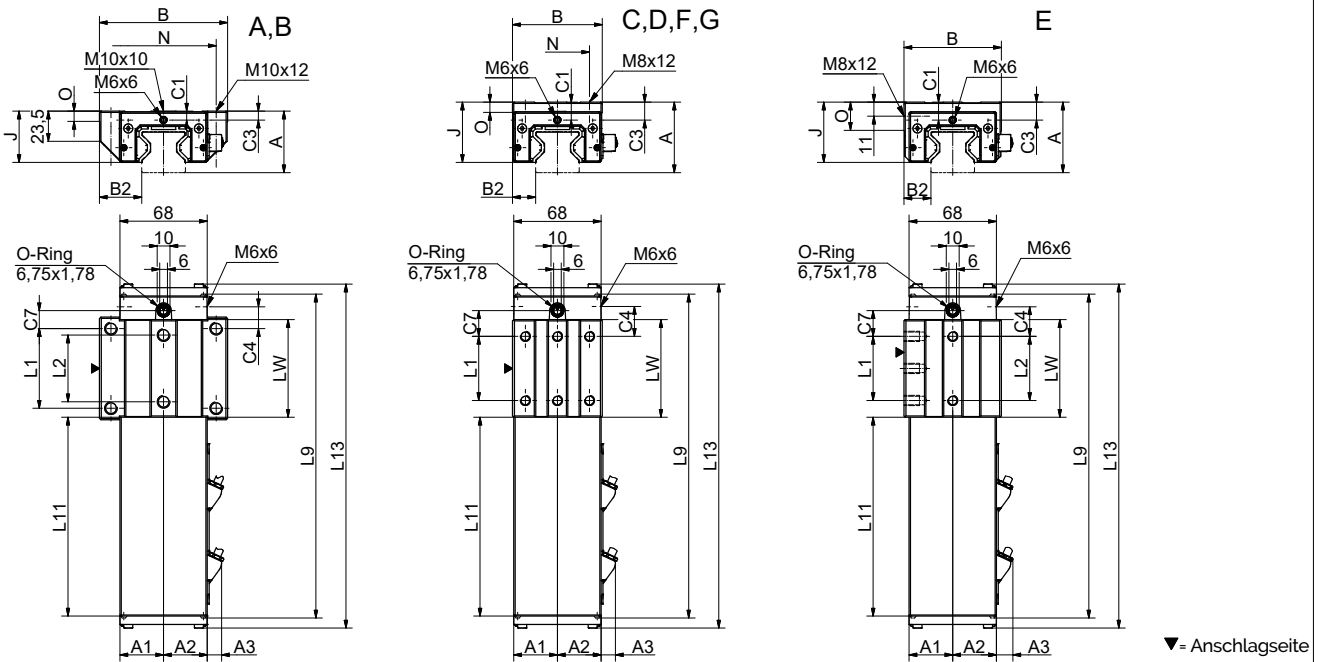
AMSABS 3L W 35 Masszeichnungen
