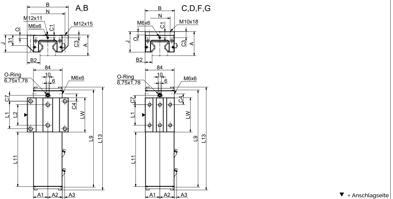
AMSABS 3L W 45 Masszeichnungen
