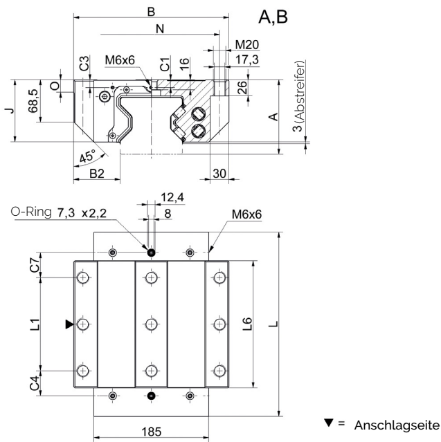
MR W 100 Masszeichnungen
