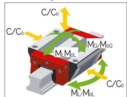
BM WR 15 Tragzahlen
