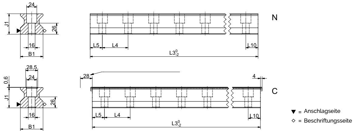
AMS 3B S 55 Masszeichnungen
