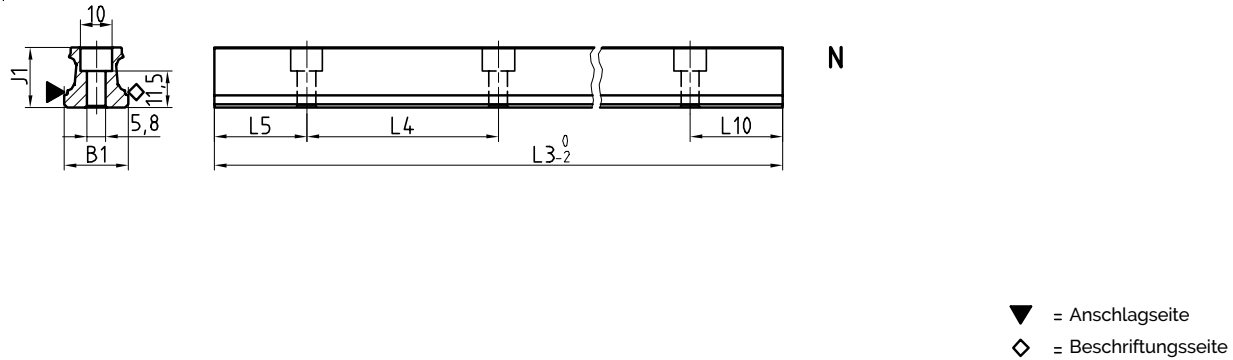
AMS 4B S 20 Masszeichnungen
