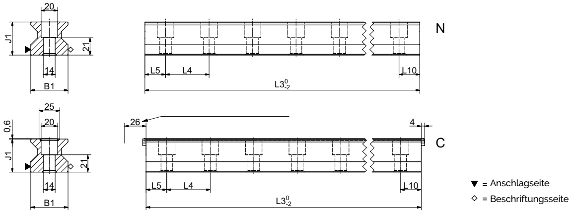
AMS 3B S 45 Masszeichnungen
