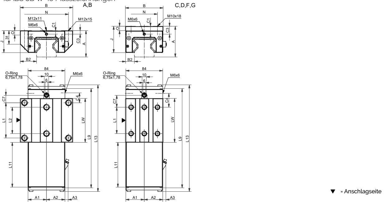
AMSABS 3B W 45 Masszeichnungen
