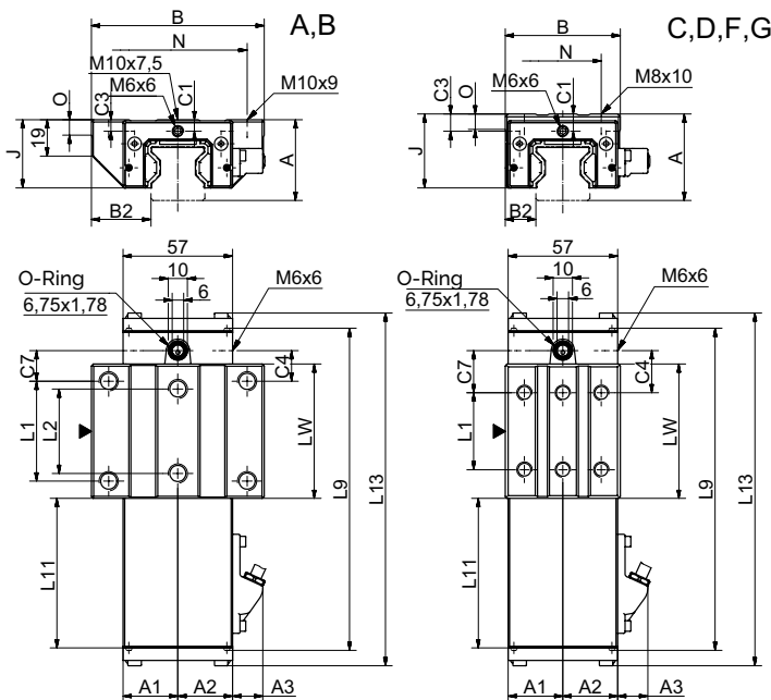
AMS 3B W 30 Masszeichnungen
