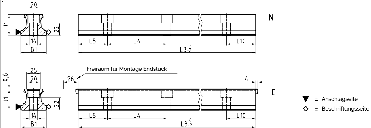
AMS 4B S 45 Masszeichnungen
