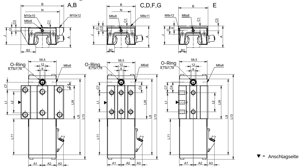
AMS 4B W 30 Masszeichnungen
