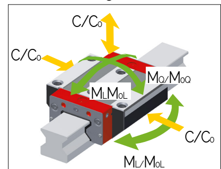
AMS 4B W 45 Tragzahlen
