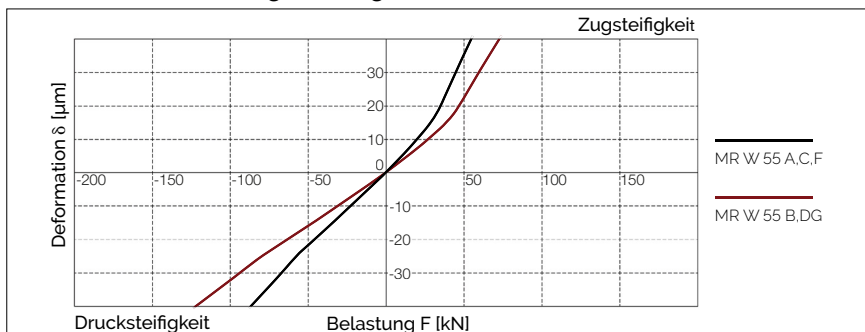
AMSABS 3B W 55 Steifigkeitsdiagramm
