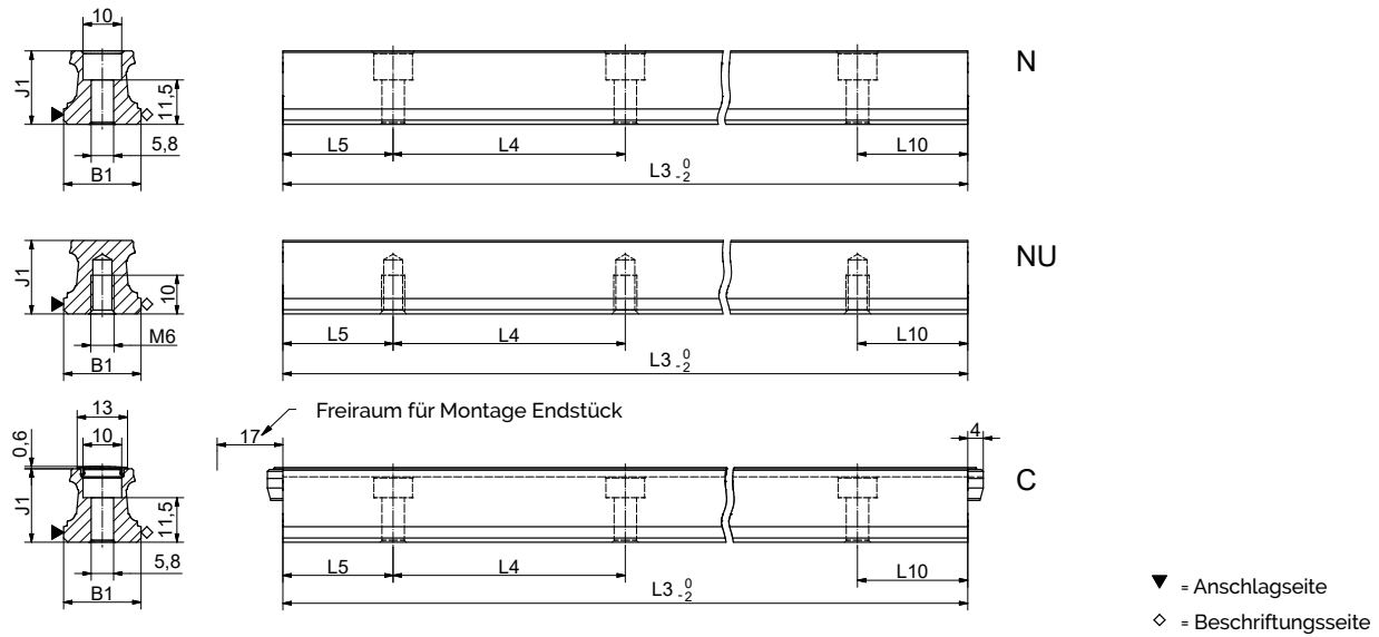
BM S 20 Masszeichnungen
