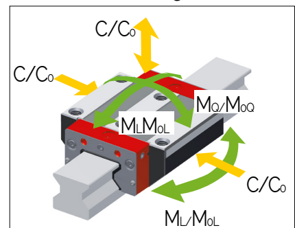
AMSABS 3B W 35 Tragzahlen
