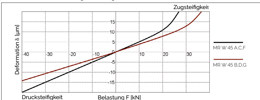
AMSABS 3B W 45 Steifigkeitsdiagramm
