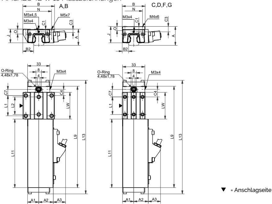
AMSABS 4B W 15 Masszeichnungen
