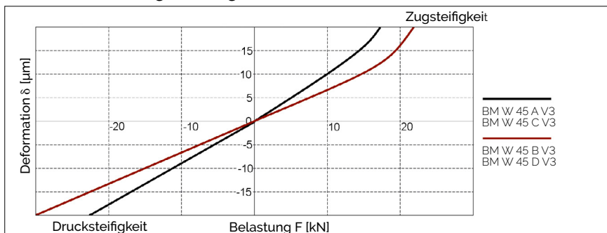
AMS 4B W 45 Steifigkeitsdiagramm
