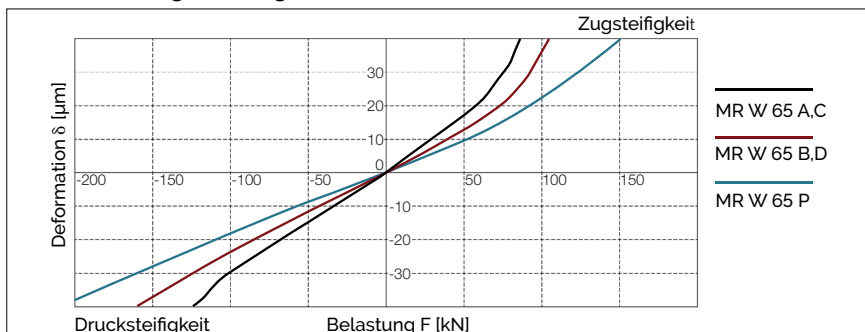
MR W 65 Steifigkeitsdiagramm
