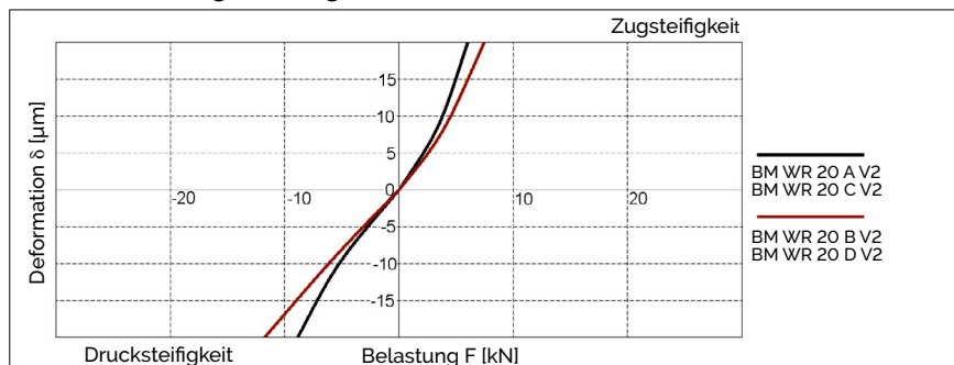
BM WR 20 Steifigkeitsdiagramm
