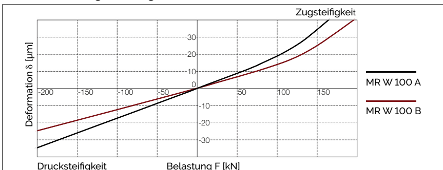
MR W 100 Steifigkeitsdiagramm
