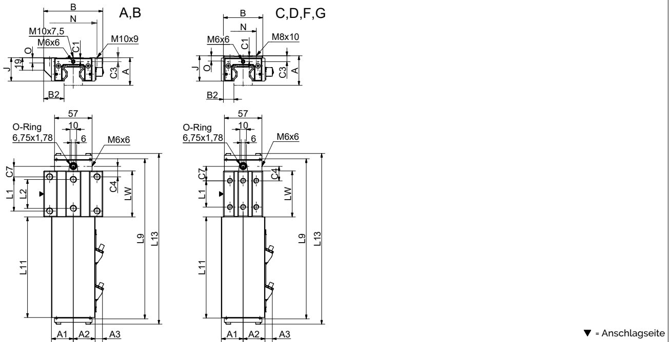
AMSABS 3L W 30 Masszeichnungen
