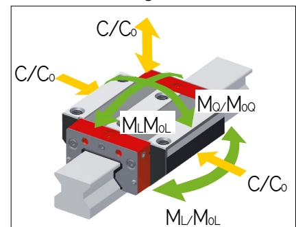
AMS 3B W 30 Tragzahlen
