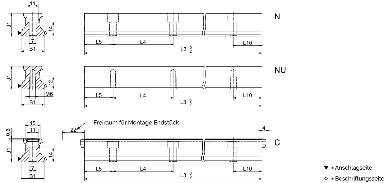
BM S 25 Masszeichnungen
