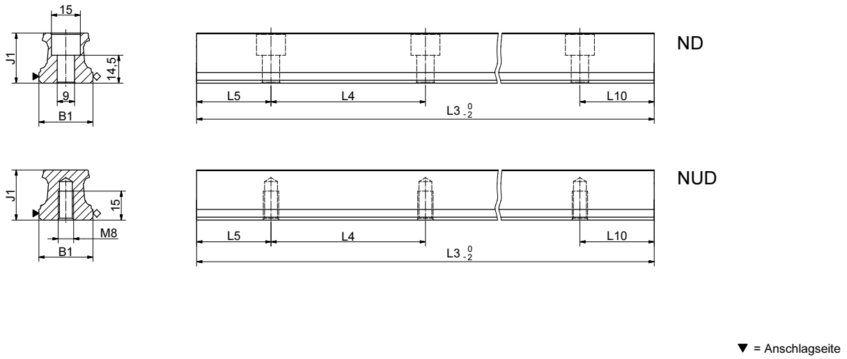
BM SR 30 Masszeichnungen
