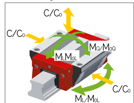
BM W 20 Tragzahlen
