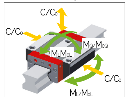
AMSABS 3B W 65 Tragzahlen
