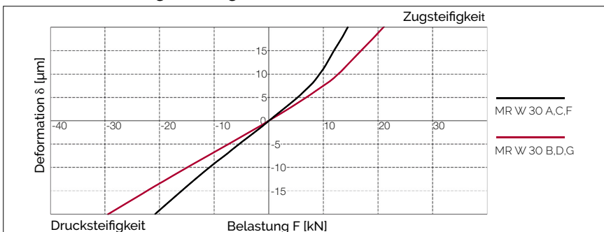
AMS 3B W 30 Steifigkeitsdiagramm
