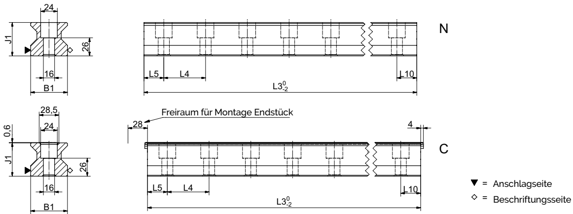
AMSABS 3B S 55 Masszeichnungen
