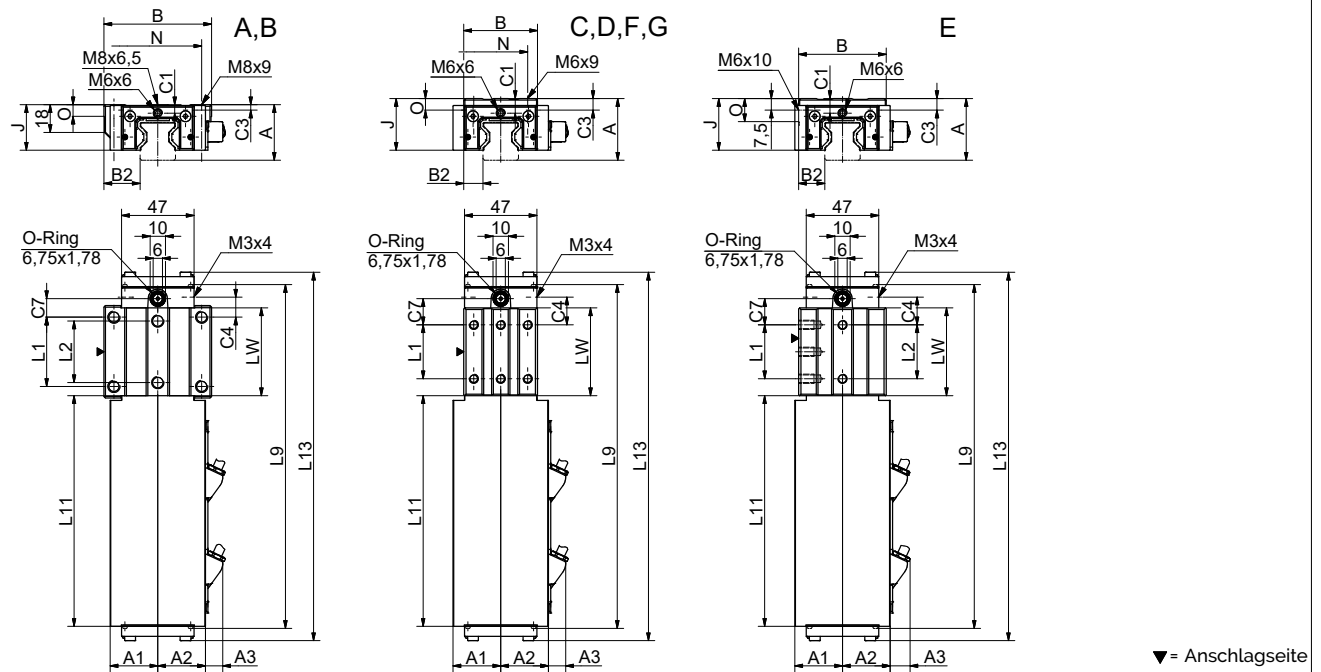
AMSABS 3L W 25 Masszeichnungen
