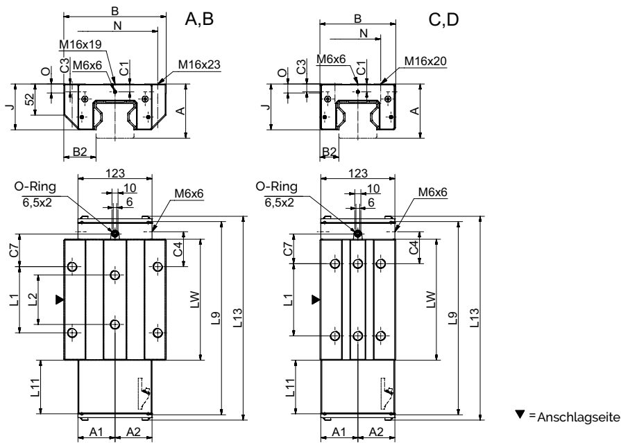
AMS 3B W 65 Masszeichnungen
