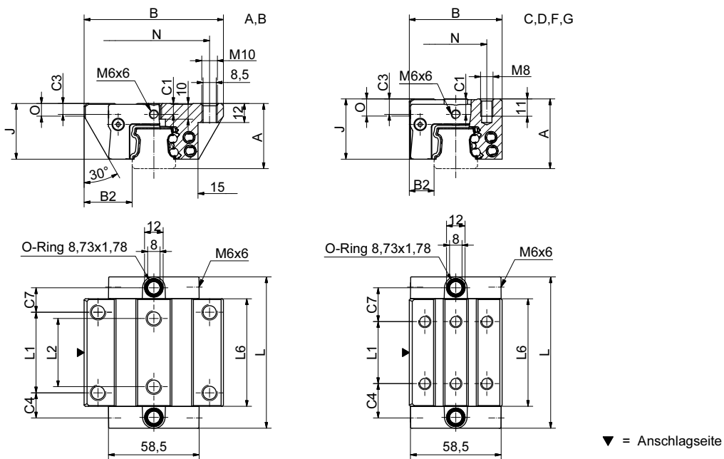
BM WR 30 Masszeichnungen
