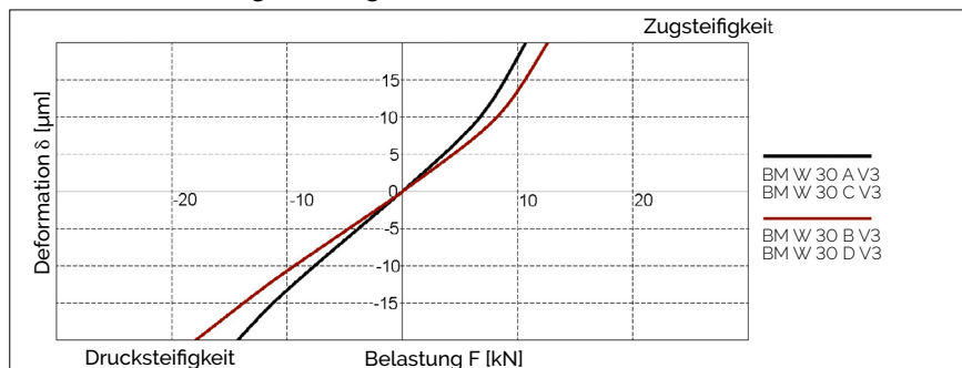
AMS 4B W 30 Steifigkeitsdiagramm
