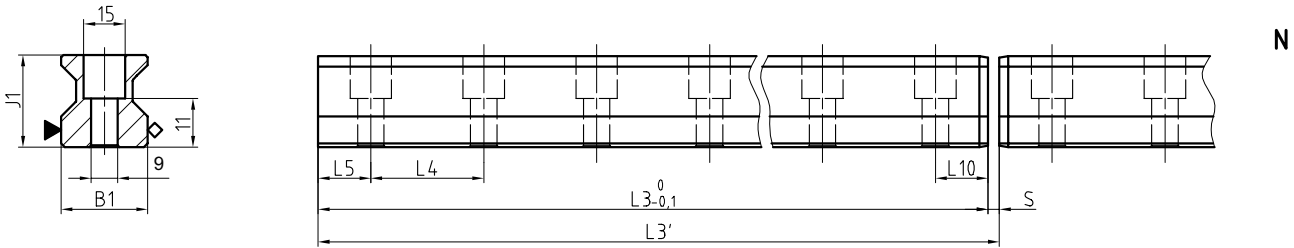
AMSABS 3L S 30 Masszeichnungen
