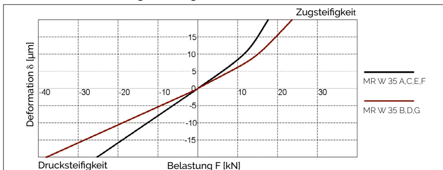
AMSABS 3B W 35 Steifigkeitsdiagramm
