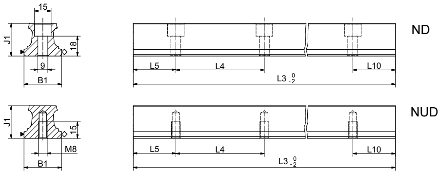
BM SR 35 Masszeichnungen
