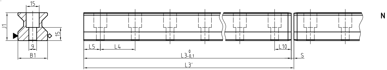
AMSABS 3L S 35 Masszeichnungen
