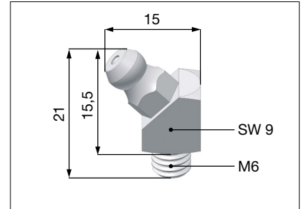
Schmiernippel SN 6-45 Kegelschmiernippel 45°
