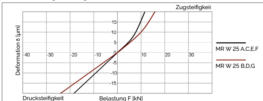
MR W 25 Steifigkeitsdiagramm
