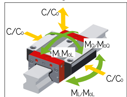
AMS 4B W 20 Tragzahlen
