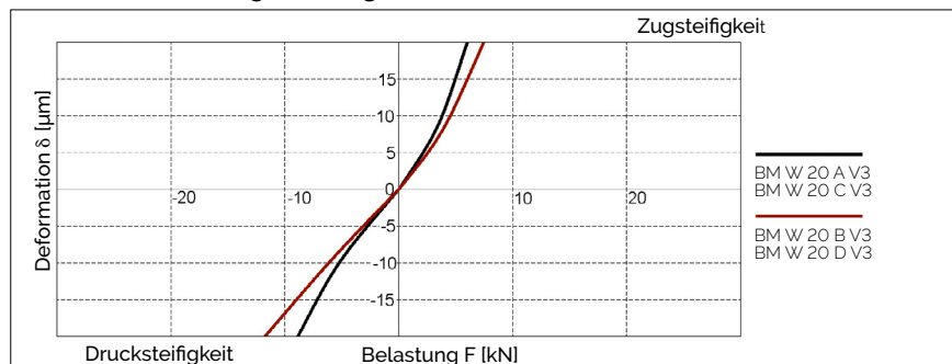
AMS 4B W 20 Steifigkeitsdiagramm
