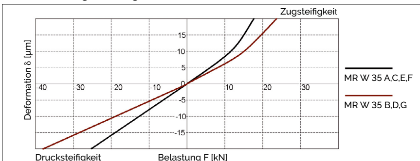
MR W 35 Steifigkeitsdiagramm
