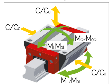
AMSABS 4B W 15 Tragzahlen
