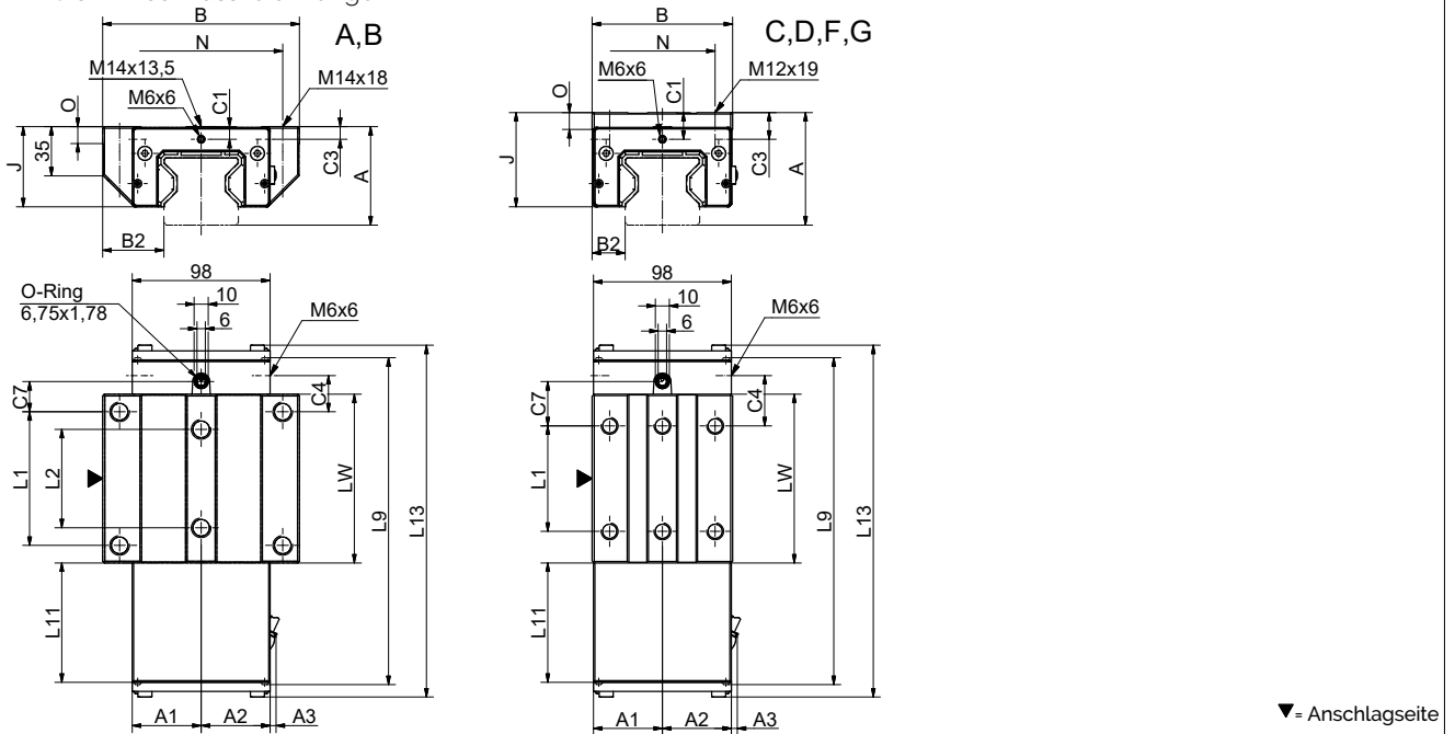
AMS 3B W 55 Masszeichnungen
