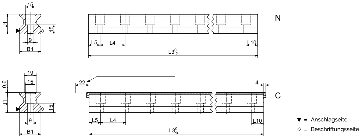
AMS 3B S 35 Masszeichnungen
