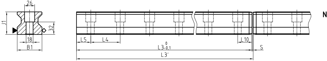
AMSABS 3L S 65 Masszeichnungen
