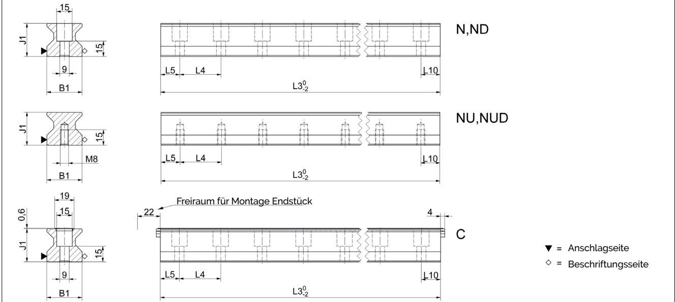
MR S 35 Masszeichnungen
