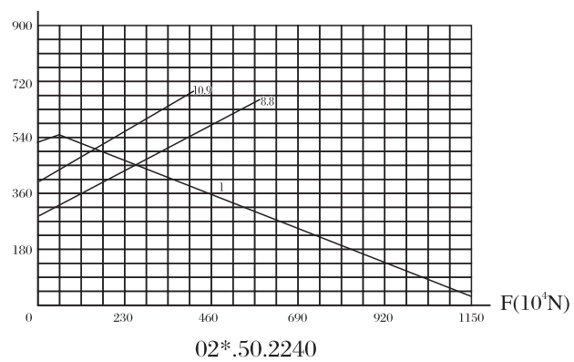
承载曲线图编号 15 Static limiting load curve 15
