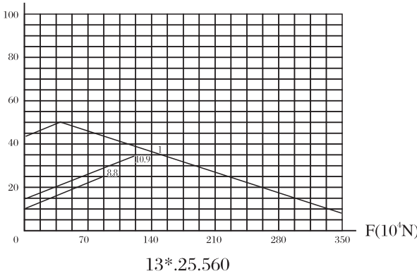
承载曲线图编号 2 Static limiting load curve 2 M(104N · m)
