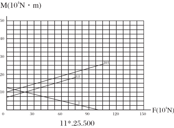
承载曲线图编号 1 Static limiting load curve 1
