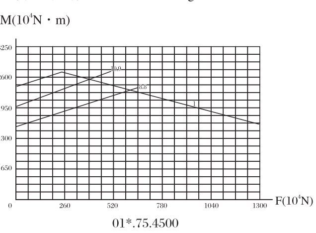
承载曲线图编号 20 Static limiting load curve 20
