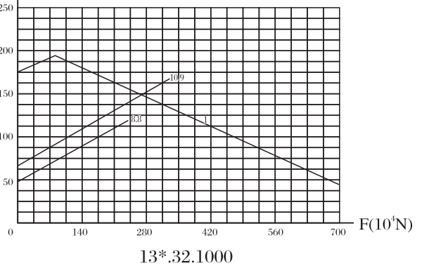
承载曲线图编号 7 Static limiting load curve 7 M(104N · m)
