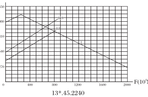
承载曲线图编号 15 Static limiting load curve 15 M(10 4 N · m)
