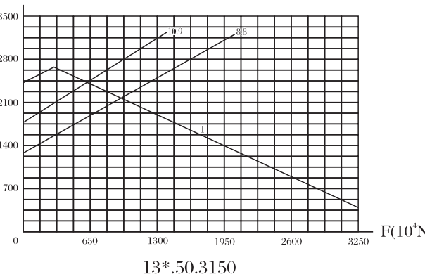
承载曲线图编号 18 Static limiting load curve 18 M(10 4 N · m)
