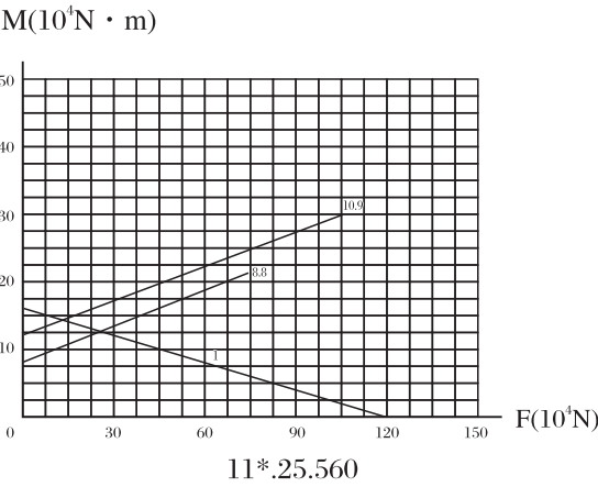
承载曲线图编号 2 Static limiting load curve 2
