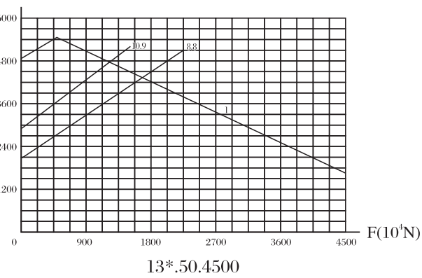
承载曲线图编号 20 Static limiting load curve 20 M(10 4 N · m)
