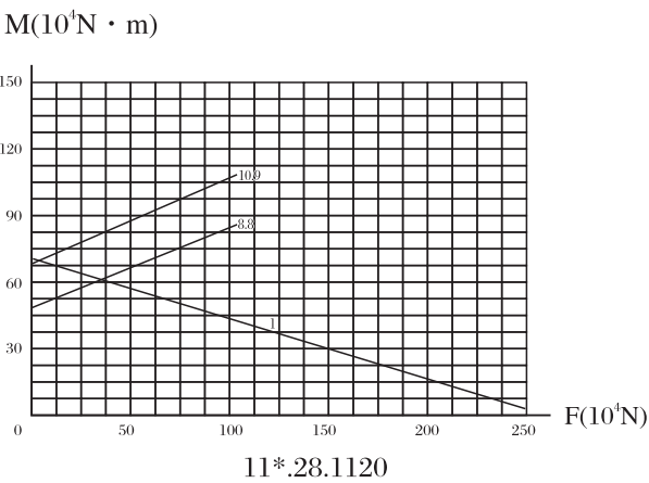
承载曲线图编号 8 Static limiting load curve 8
