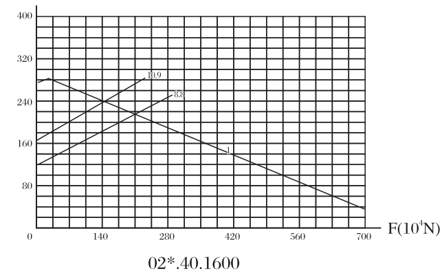
承载曲线图编号 12 Static limiting load curve 12
