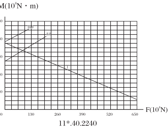
承载曲线图编号 14 Static limiting load curve 14
