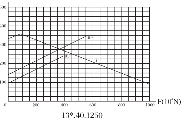
承载曲线图编号 9 Static limiting load curve 9 M(104N · m)
