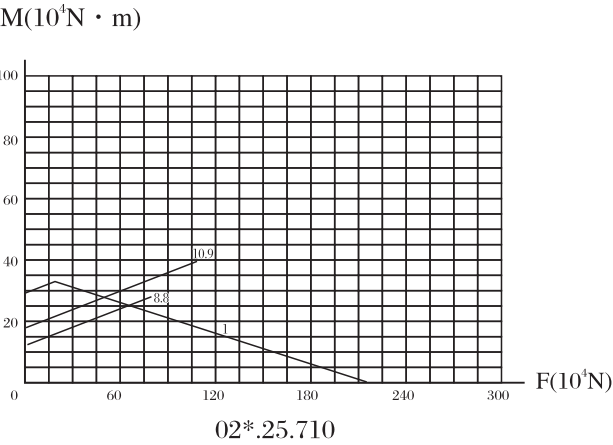
承载曲线图编号 4 Static limiting load curve 4
