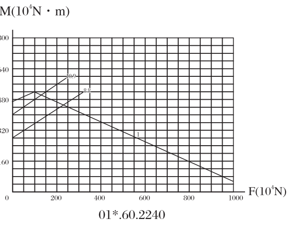
承载曲线图编号 14 Static limiting load curve 14
