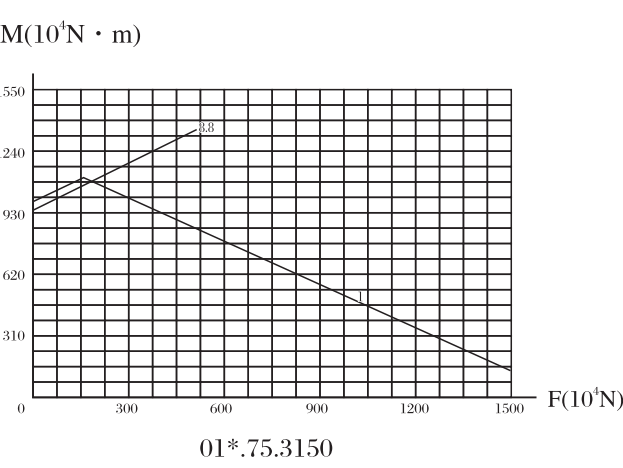
承载曲线图编号 17 Static limiting load curve 17
