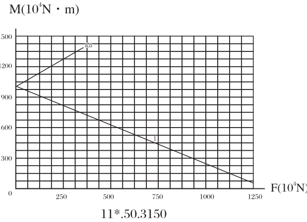
承载曲线图编号 17 Static limiting load curve 17
