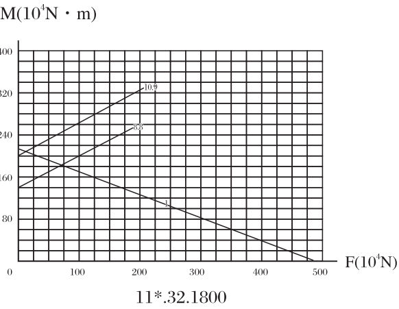
承载曲线图编号 12 Static limiting load curve 12
