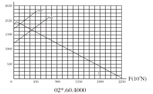
承载曲线图编号 20 Static limiting load curve 20
