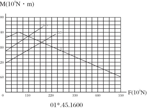
承载曲线图编号 11 Static limiting load curve 11
