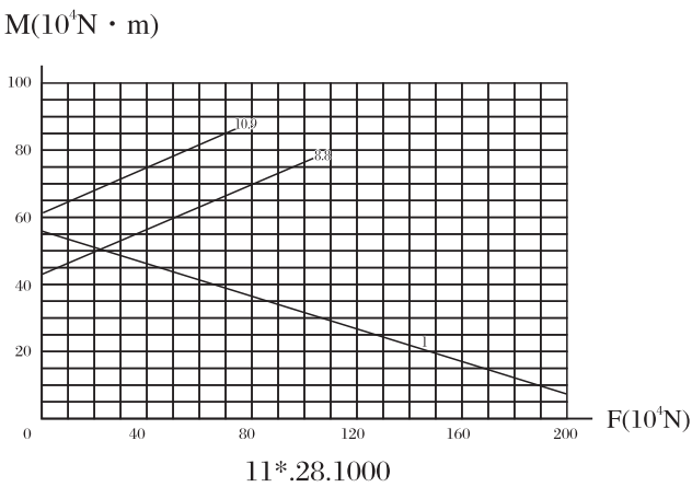
承载曲线图编号 7 Static limiting load curve 7
