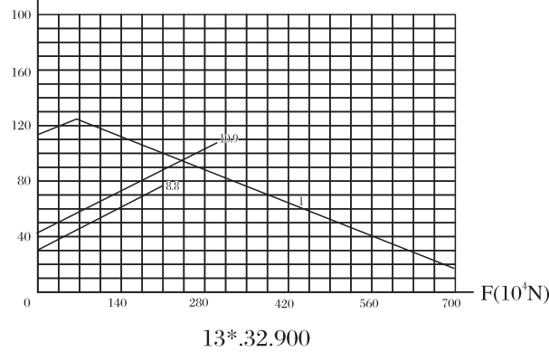
承载曲线图编号 6 Static limiting load curve 6 M(104N · m)
