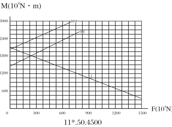
承载曲线图编号 20 Static limiting load curve 20
