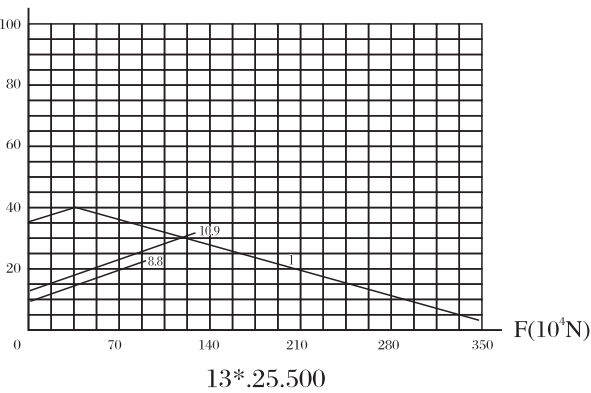
承载曲线图编号 1 Static limiting load curve 1 M(104N · m)
