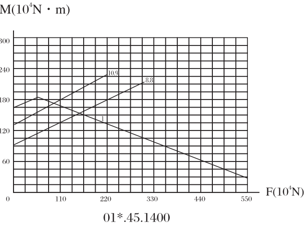
承载曲线图编号 10 Static limiting load curve 10
