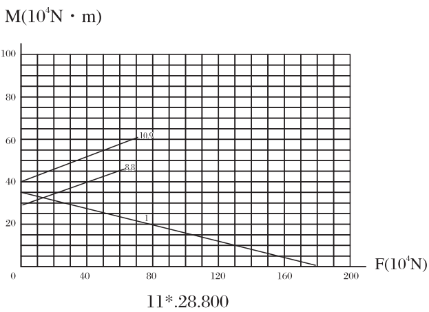
承载曲线图编号 5 Static limiting load curve 5
