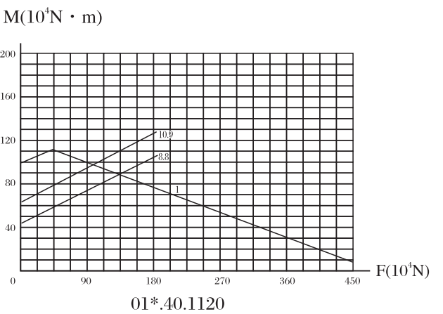
承载曲线图编号 8 Static limiting load curve 8
