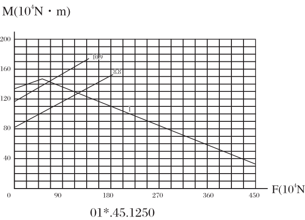
承载曲线图编号 9 Static limiting load curve 9
