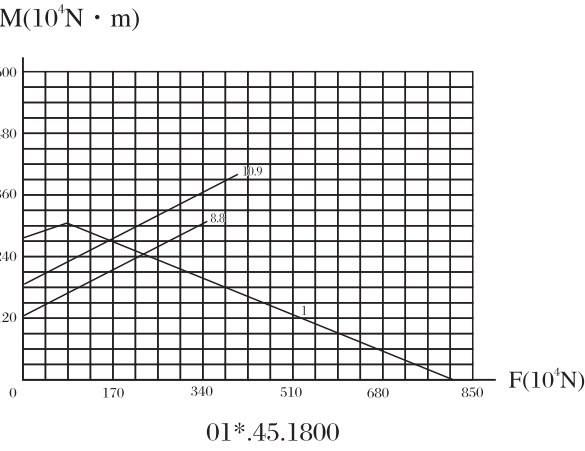
承载曲线图编号 12 Static limiting load curve 12
