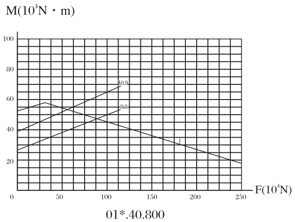
承载曲线图编号 5 Static limiting load curve 5
