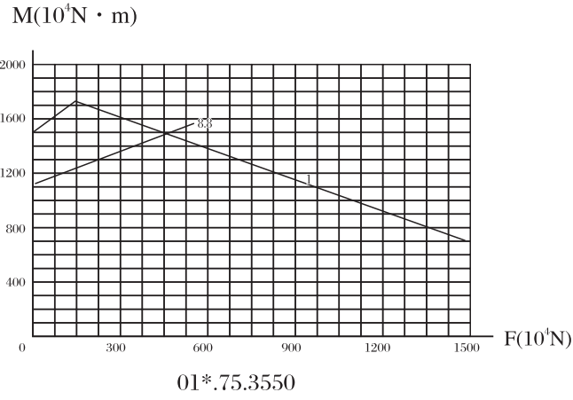
承载曲线图编号 18 Static limiting load curve 18
