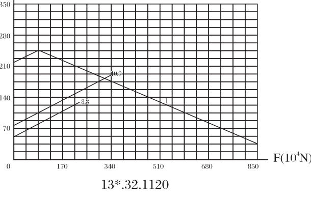
承载曲线图编号 8 Static limiting load curve 8 M(104N · m)
