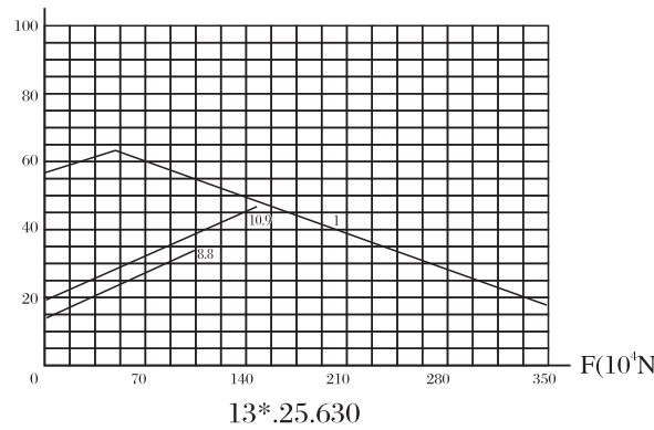
承载曲线图编号 3 Static limiting load curve 3 M(104N · m)
