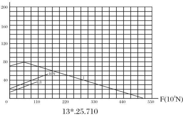
承载曲线图编号 4 Static limiting load curve 4 M(104N · m)
