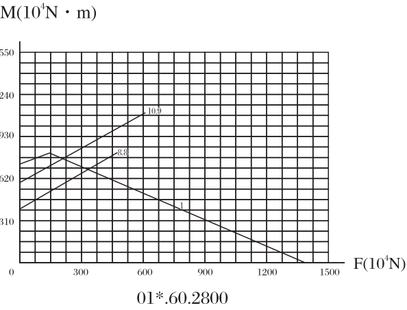
承载曲线图编号 16 Static limiting load curve 16
