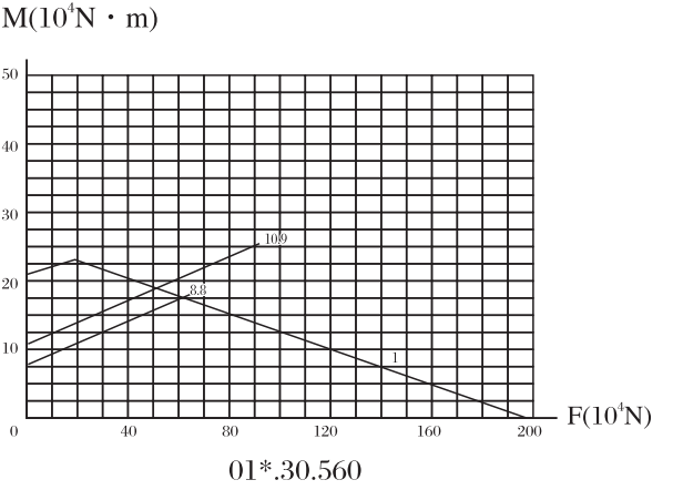
承载曲线图编号 2 Static limiting load curve 2
