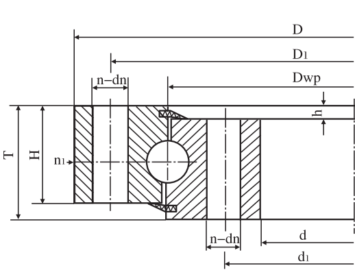
无齿式单排四点接触球轴承（010） Without Gear
