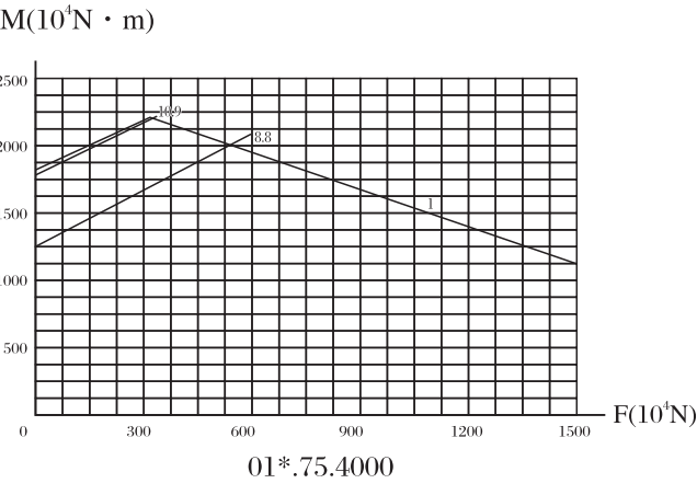
承载曲线图编号 19 Static limiting load curve 19
