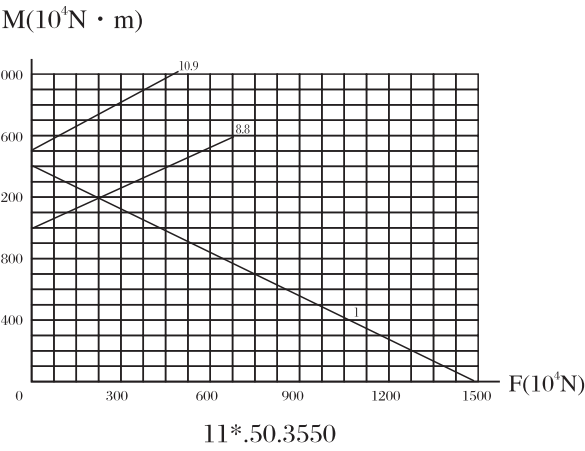
承载曲线图编号 18 Static limiting load curve 18
