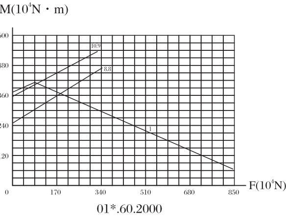
承载曲线图编号 13 Static limiting load curve 13
