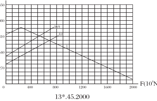
承载曲线图编号 13 Static limiting load curve 13 M(10 4 N · m)
