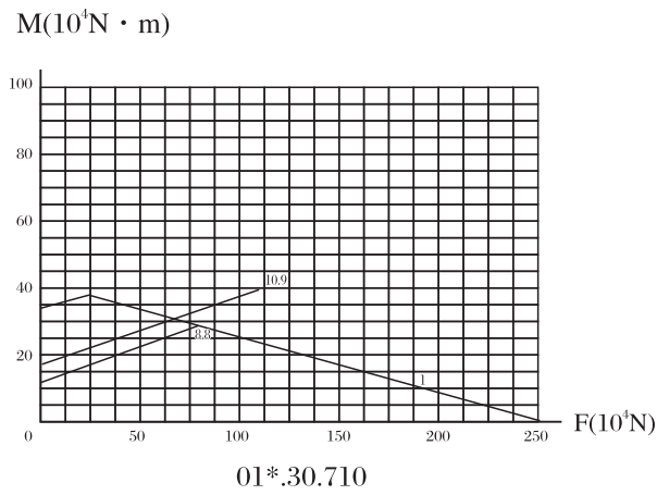
承载曲线图编号 4 Static limiting load curve 4
