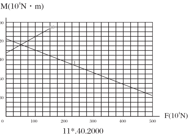
承载曲线图编号 13 Static limiting load curve 13
