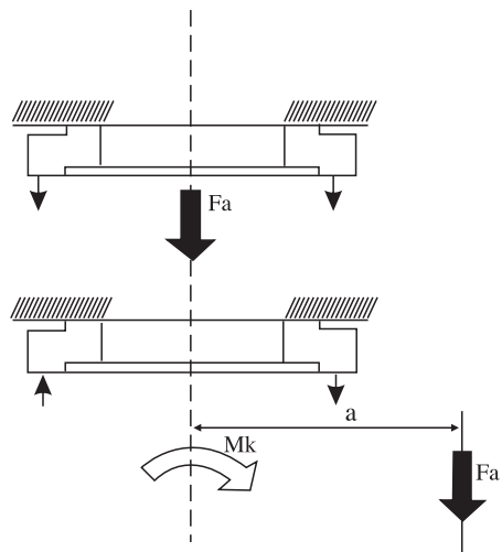
图 2：悬挂式安装 Fig. 2: Suspension installation
