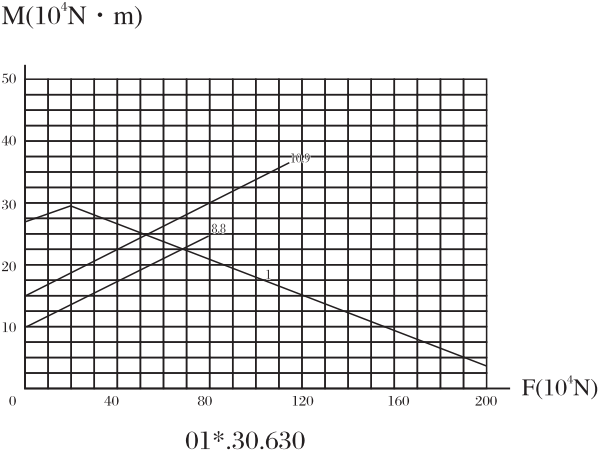
承载曲线图编号 3 Static limiting load curve 3
