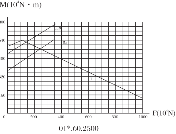
承载曲线图编号 15 Static limiting load curve 15
